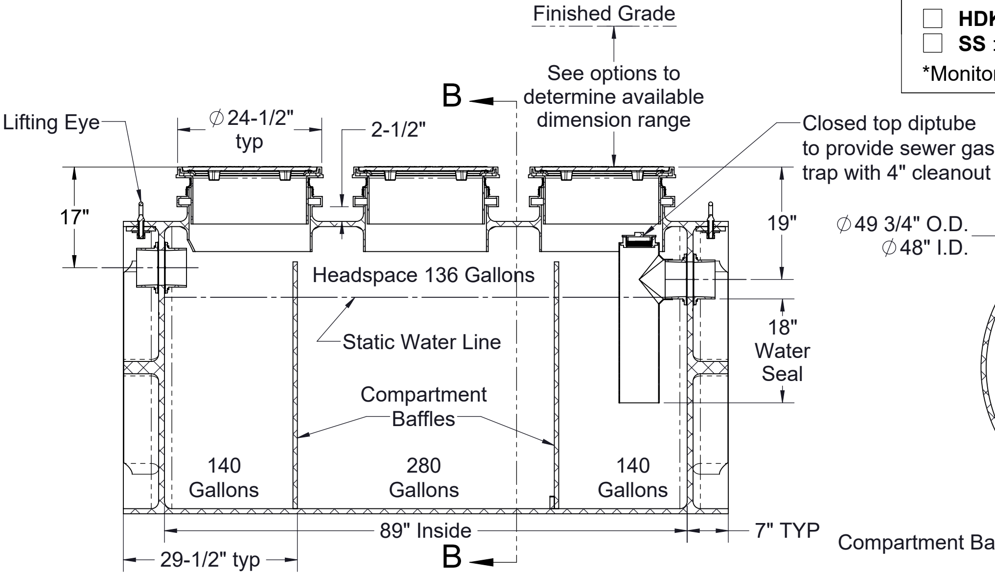
SECTION A-A
