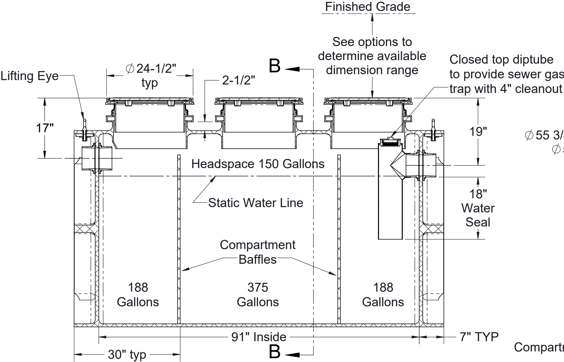
SECTION A-A
