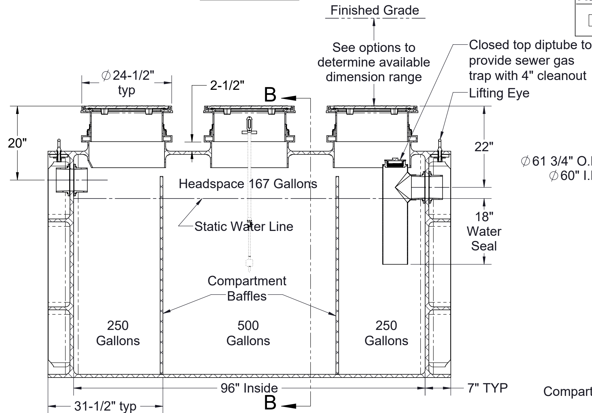
SECTION A-A
