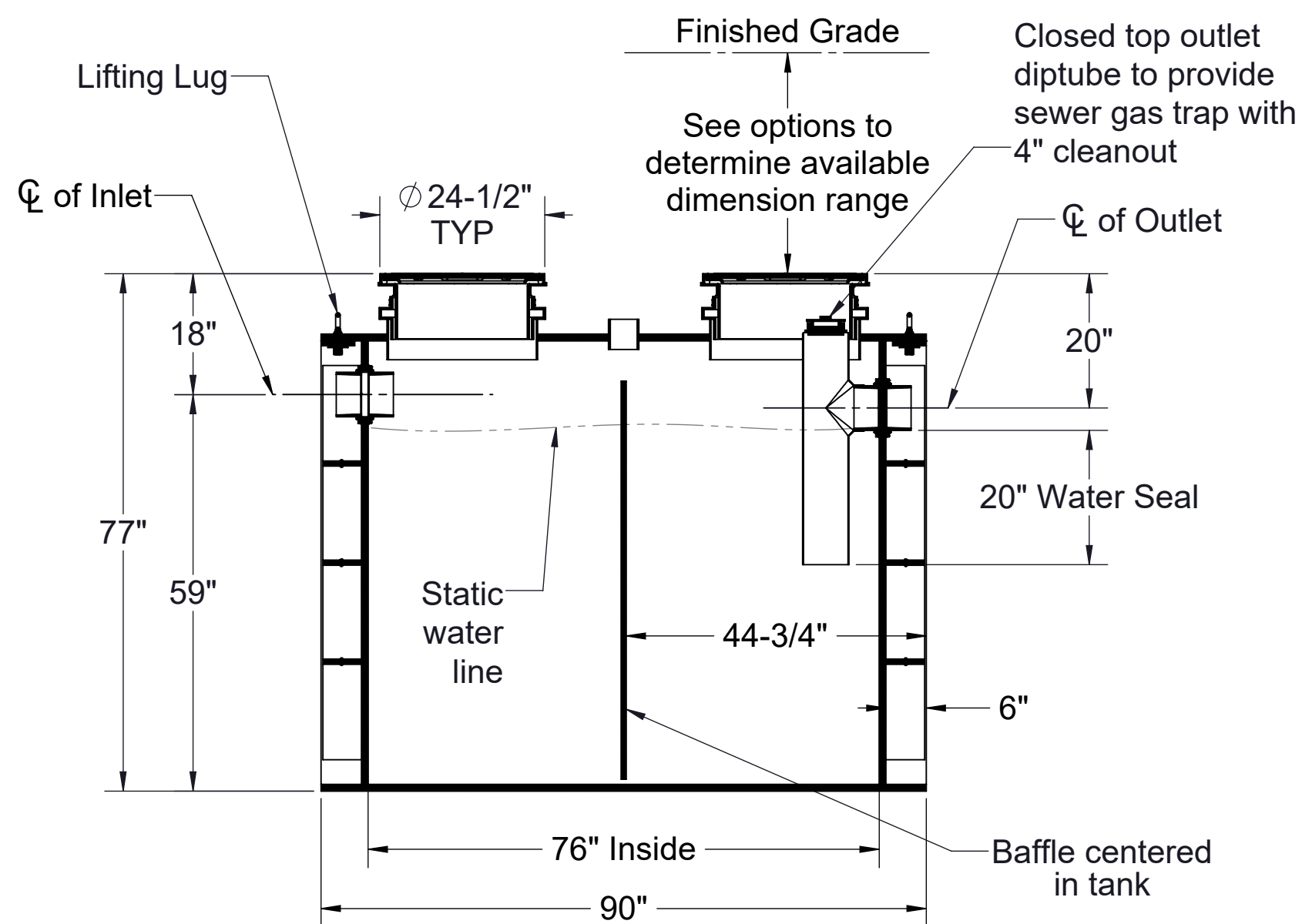
SECTION A-A
