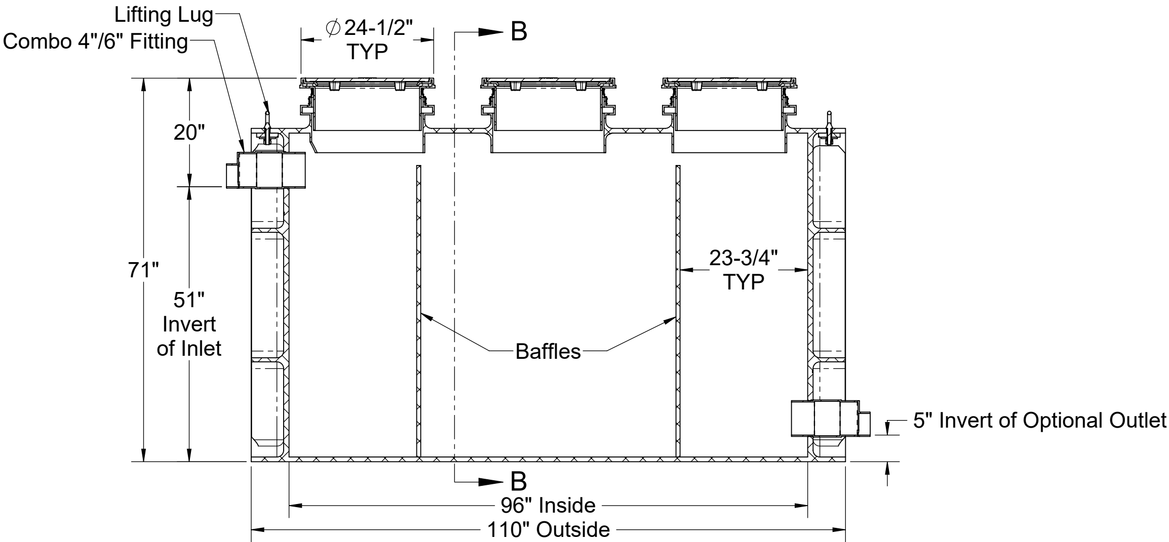
SECTION A-A
