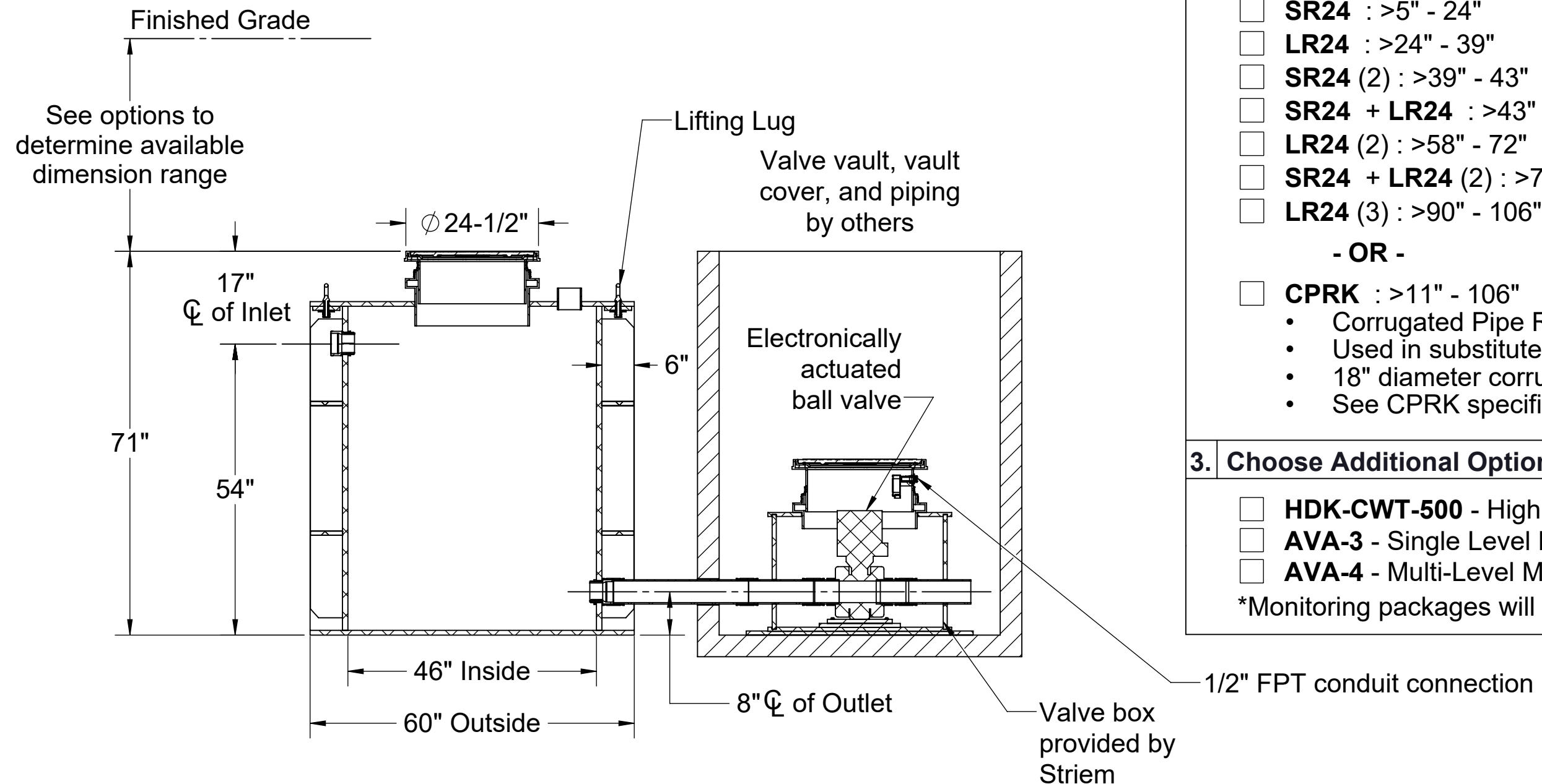
SECTION A-A
