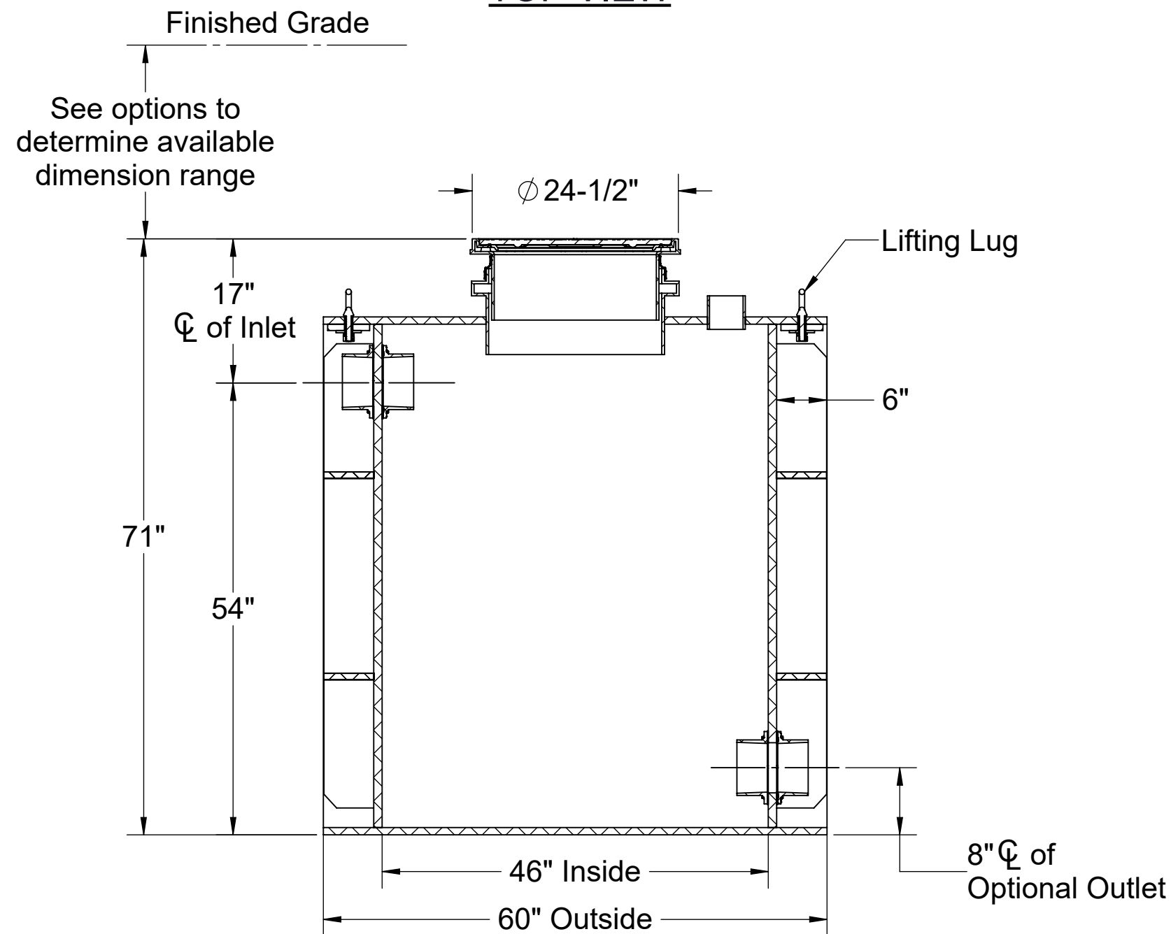
SECTION A-A
