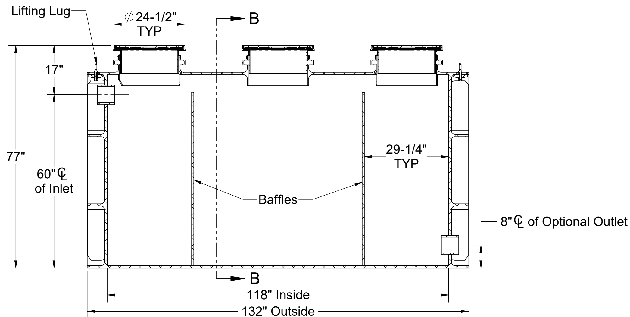
SECTION A-A
