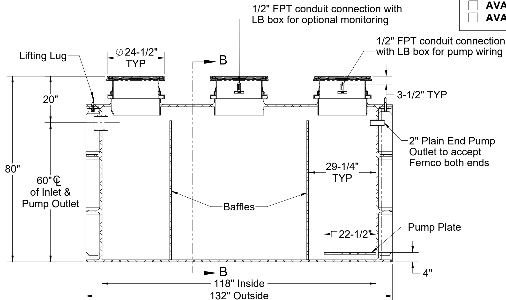
SECTION A-A
