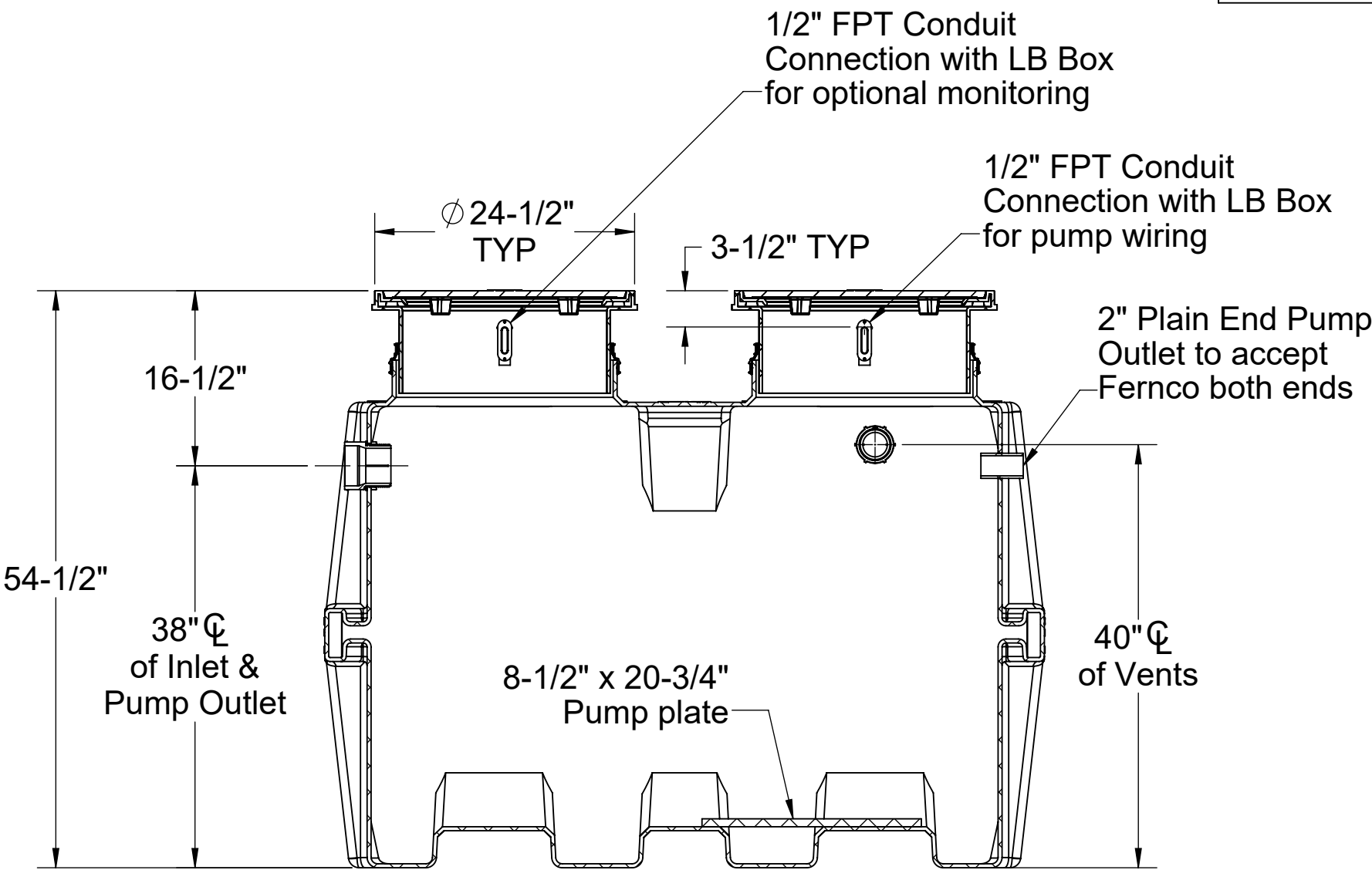
SECTION A-A
