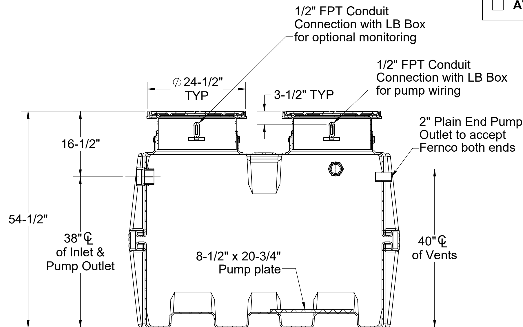
SECTION A-A
