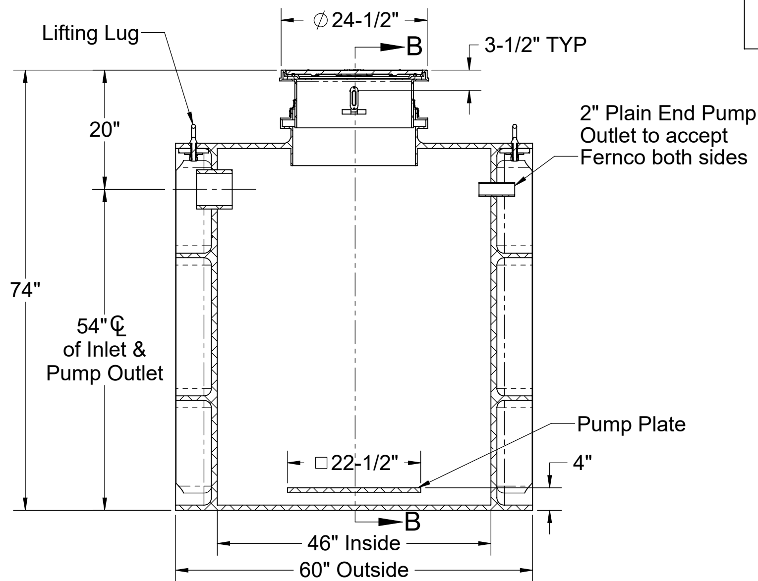
SECTION A-A
