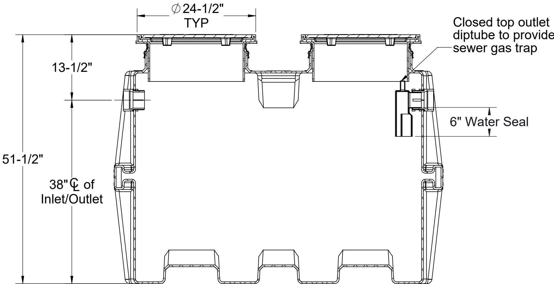
SECTION A-A
