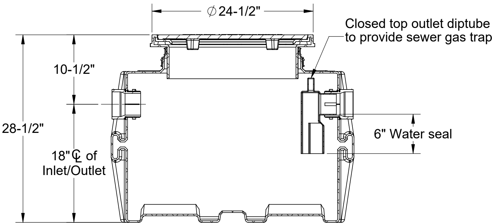
SECTION A-A
