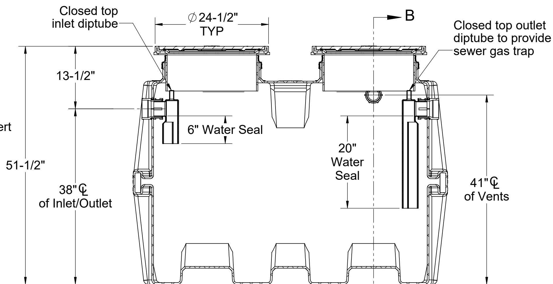
SECTION A-A
