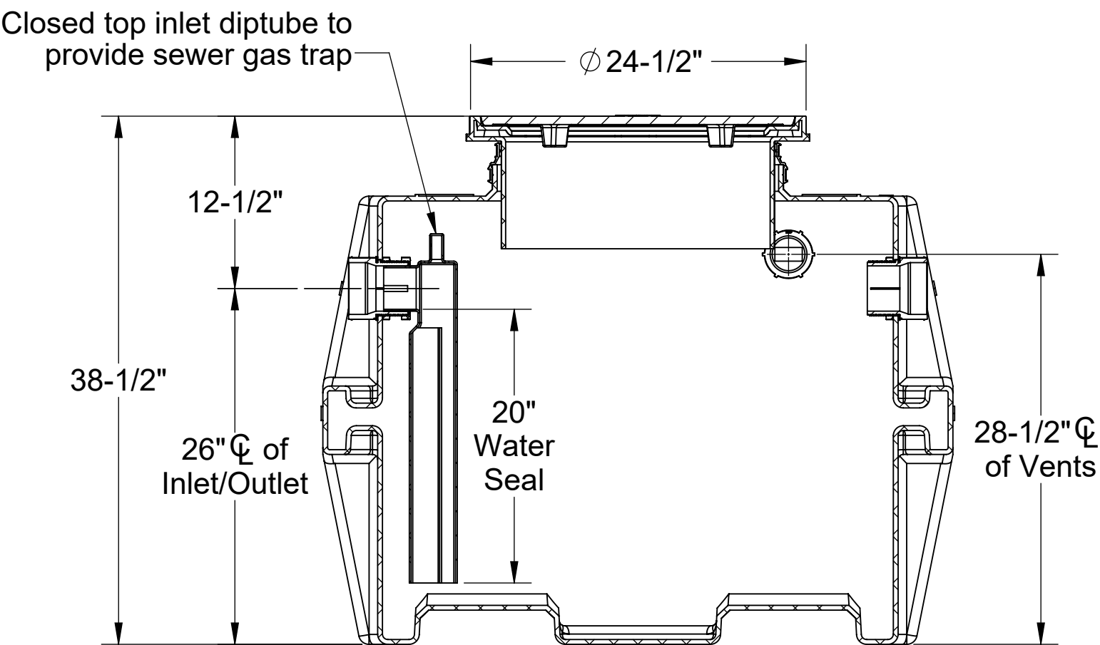
SECTION A-A
