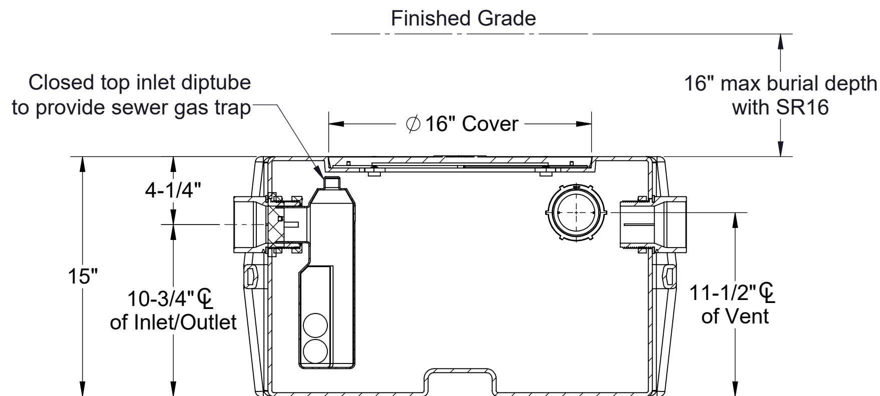
SECTION A-A
