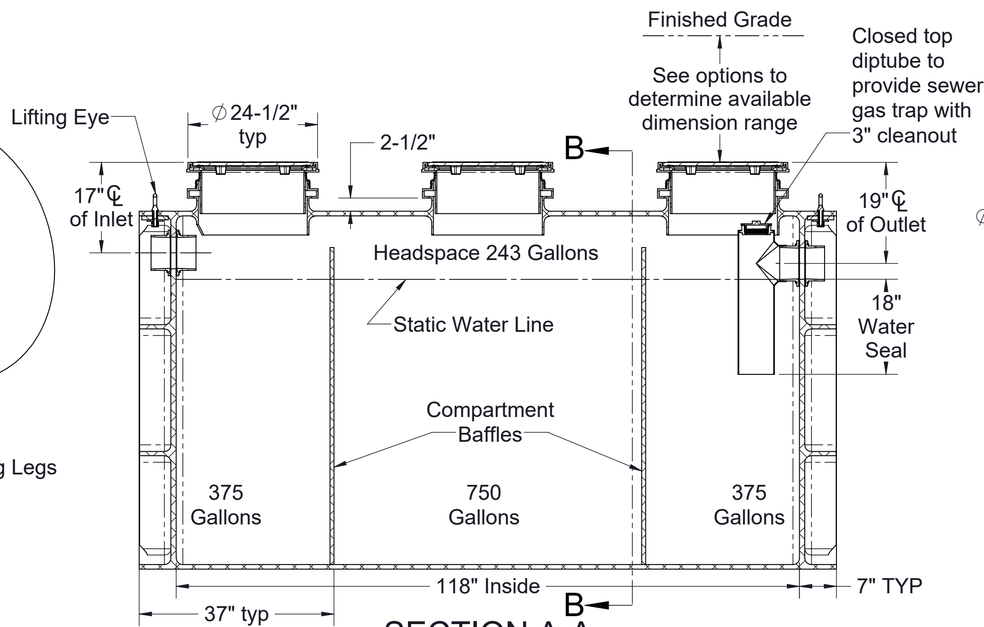
SECTION A-A
