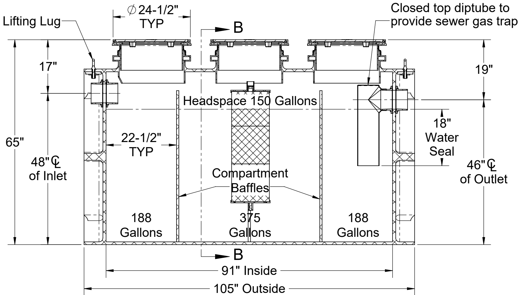
SECTION A-A
