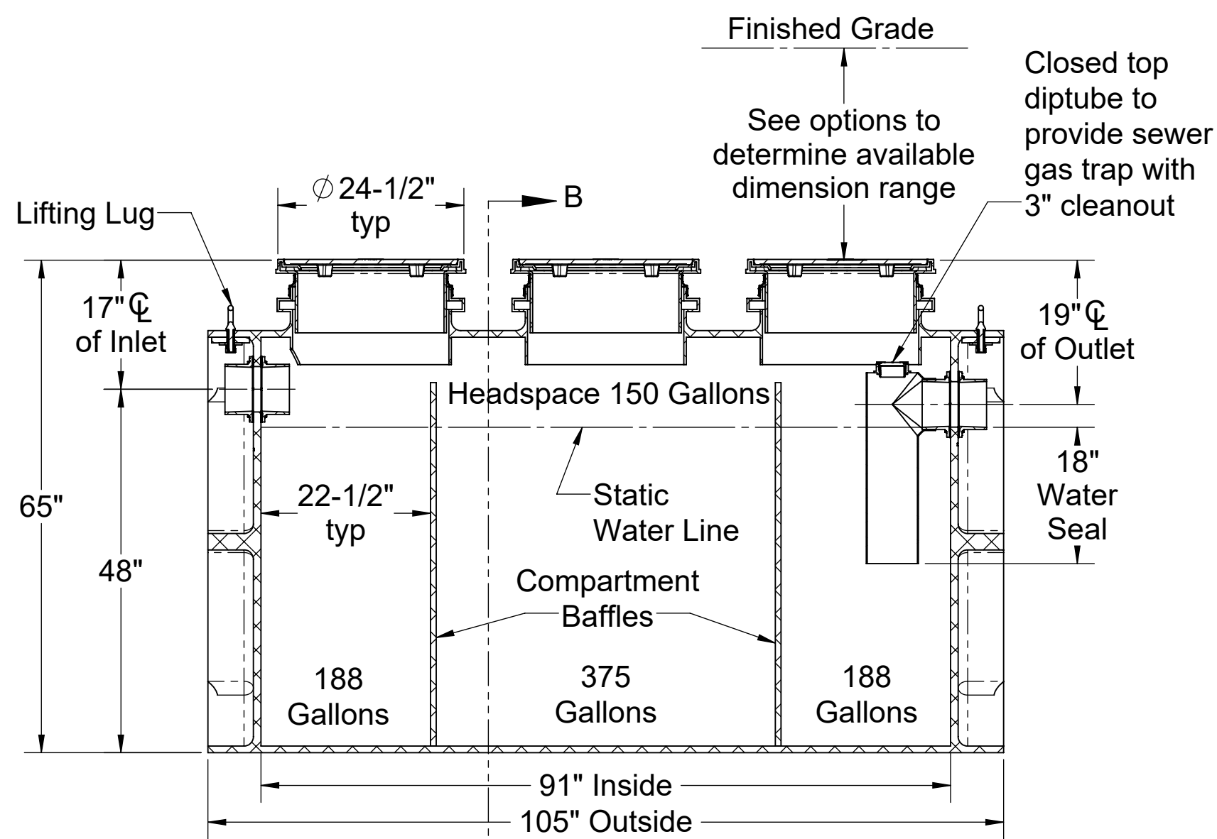
SECTION A-A
