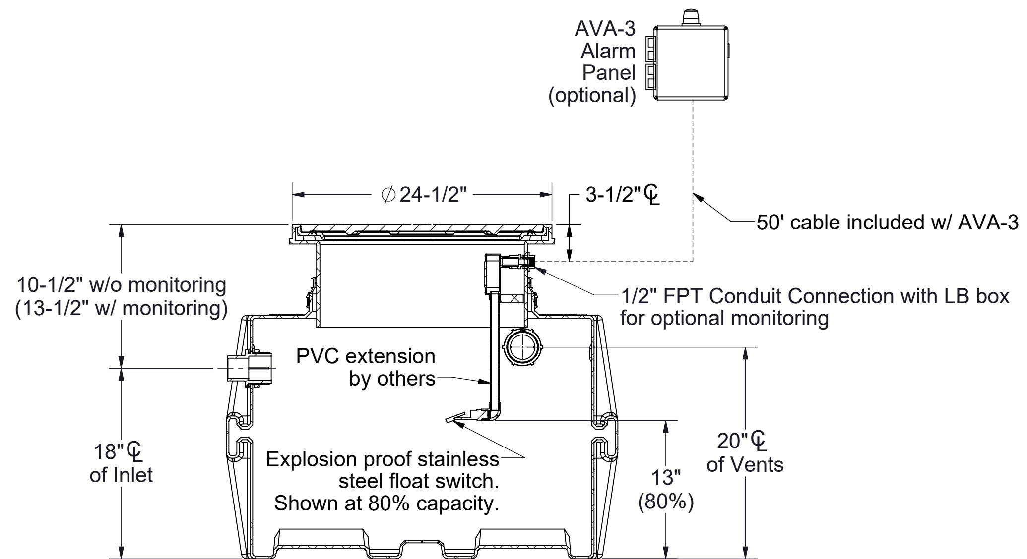
SECTION A-A
