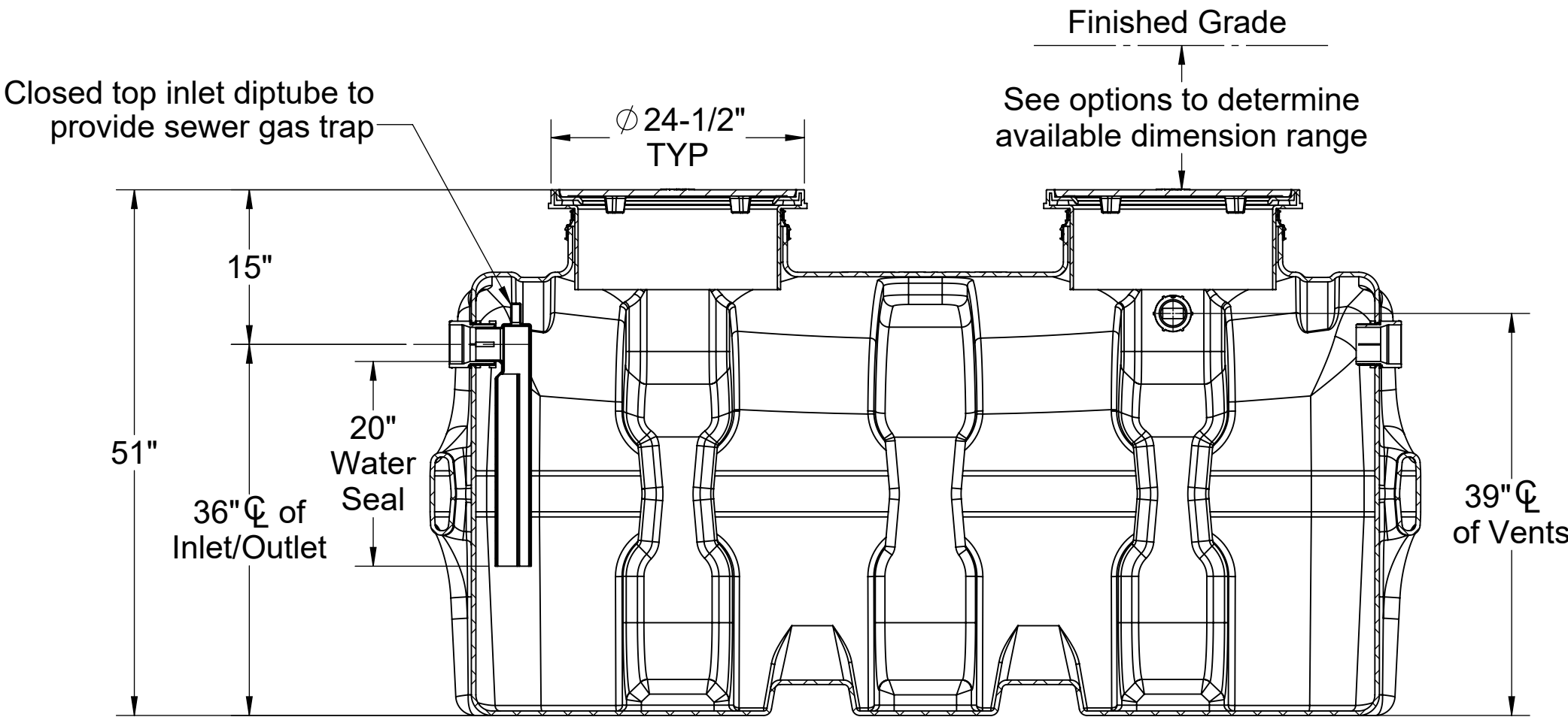
SECTION A-A
