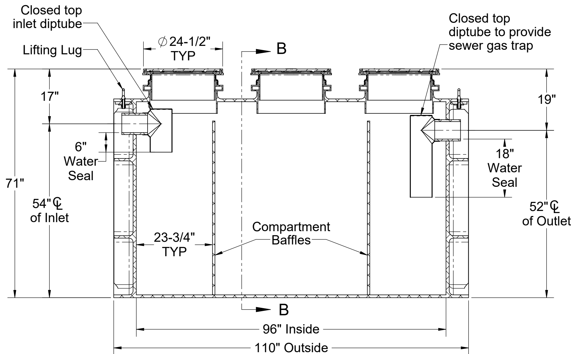
SECTION A-A
