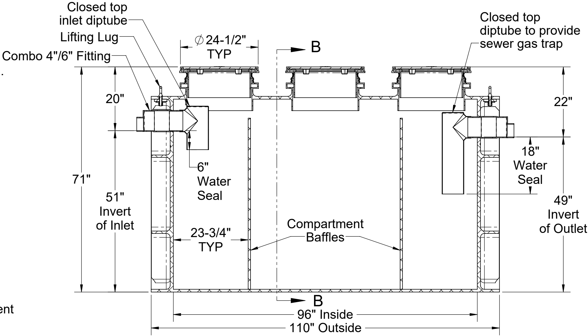
SECTION A-A
