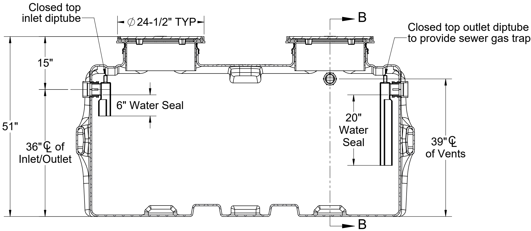
SECTION A-A
