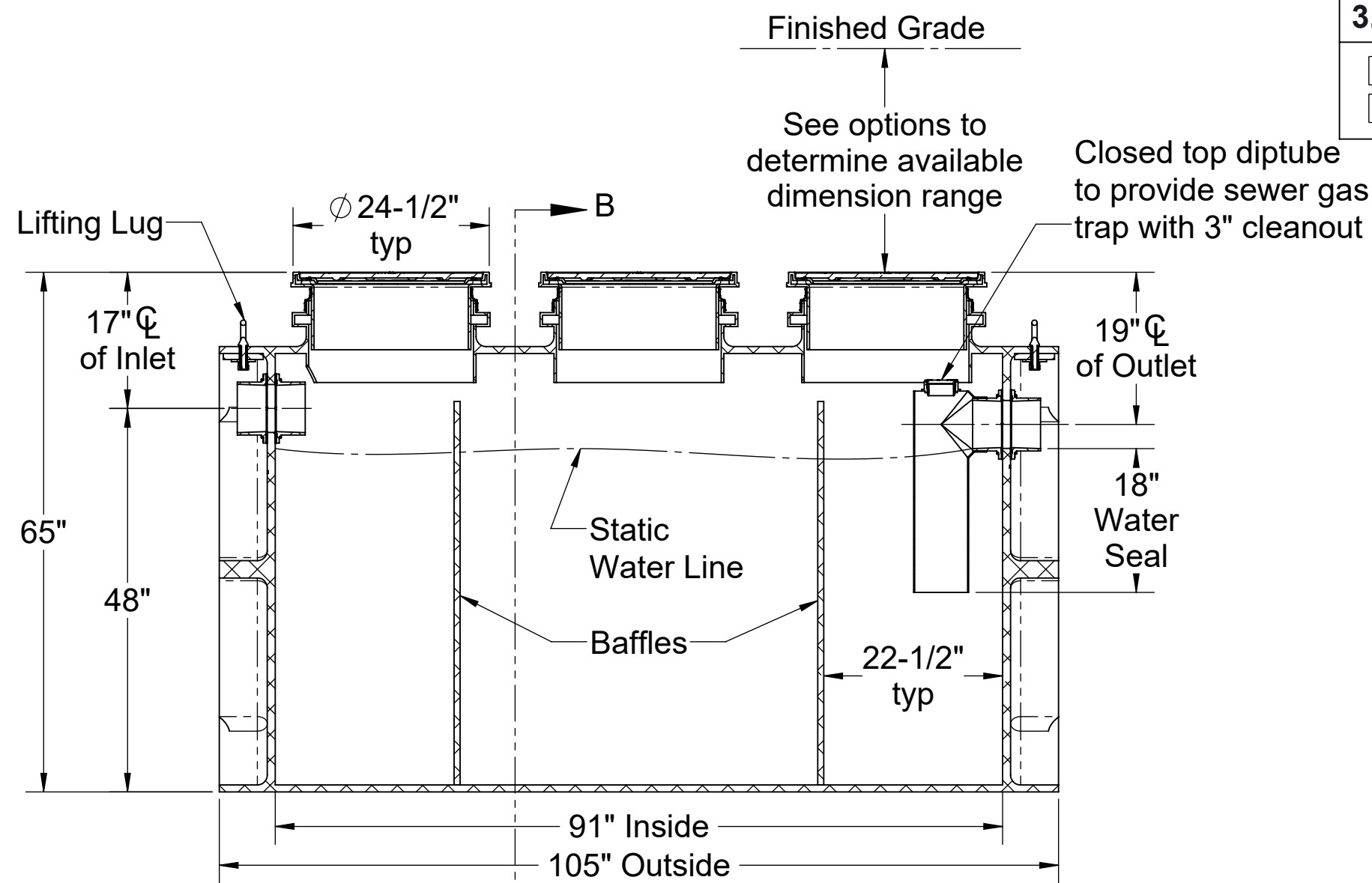
SECTION A-A
