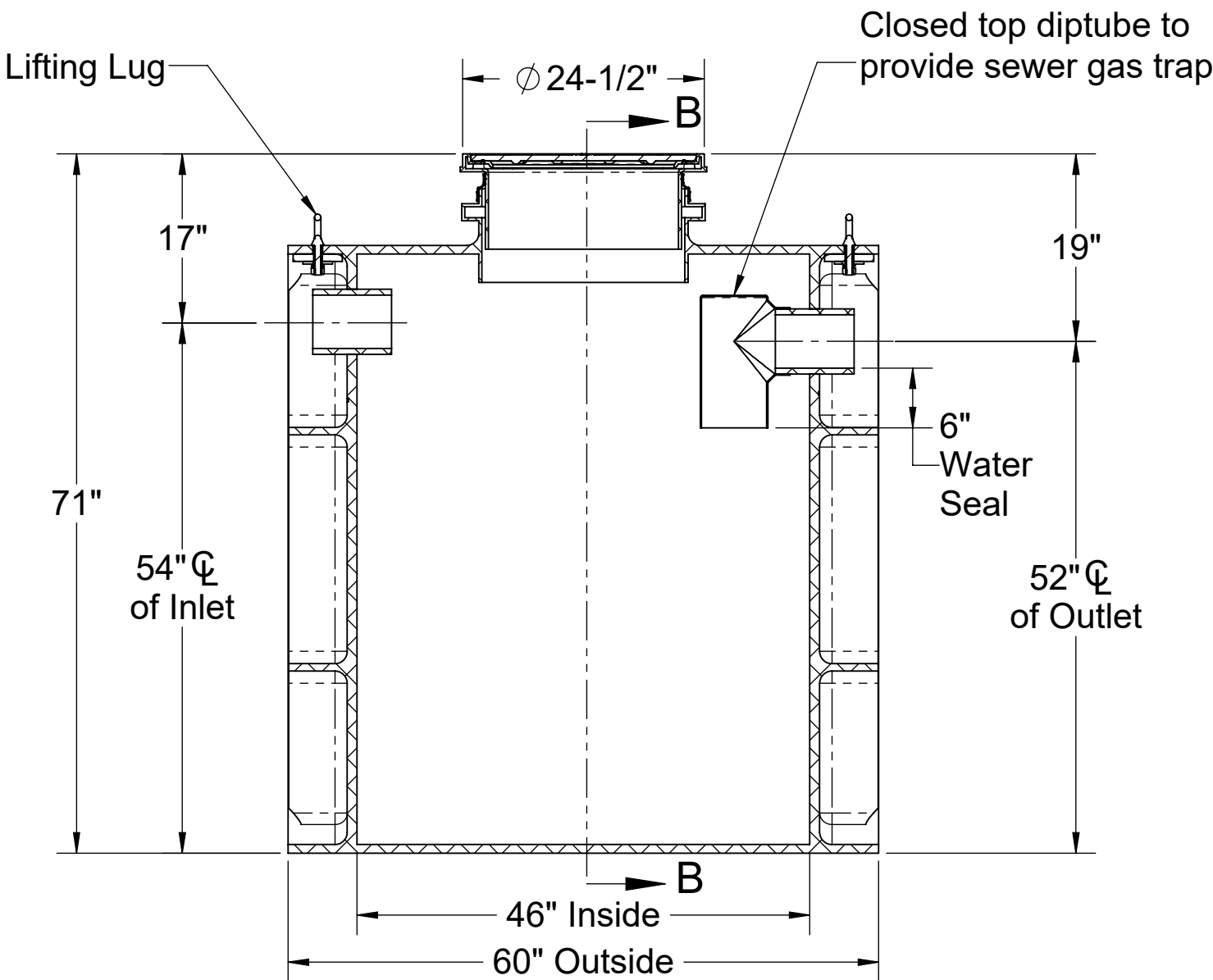
SECTION A-A
