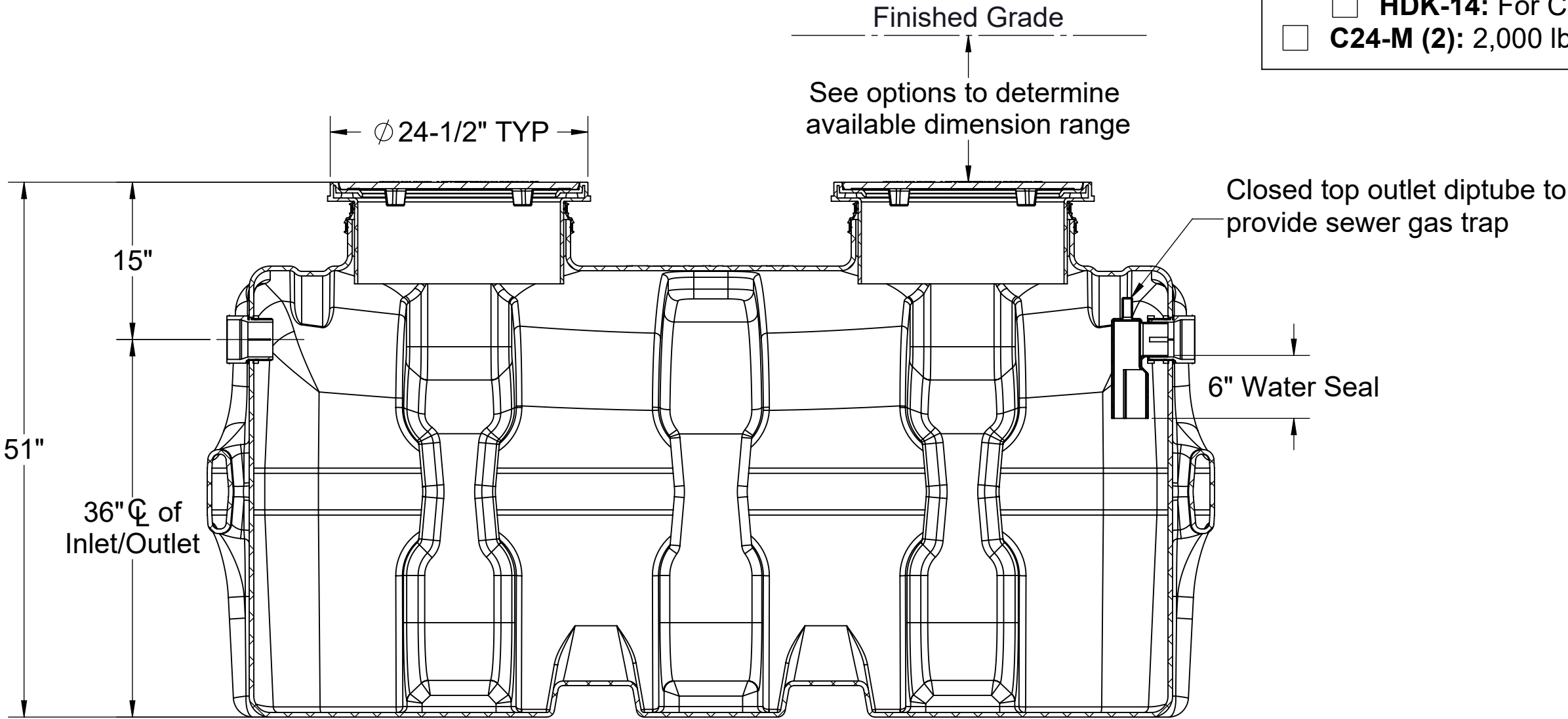
SECTION A-A
