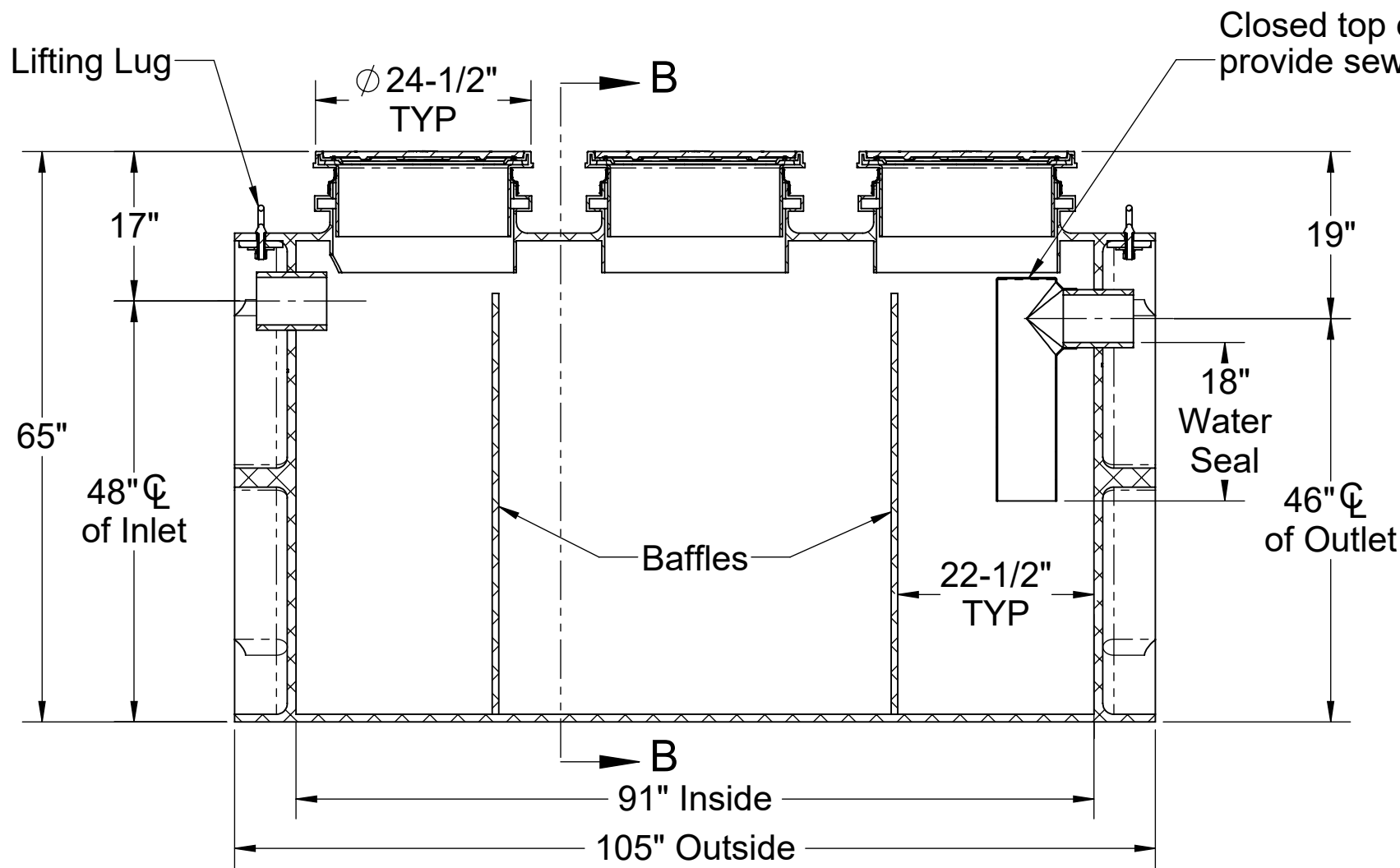
SECTION A-A
