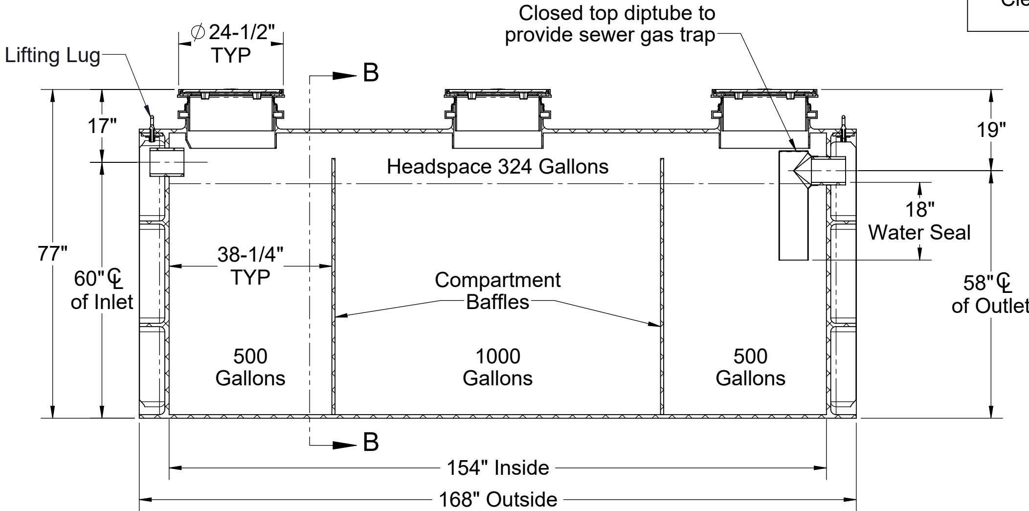
SECTION A-A
