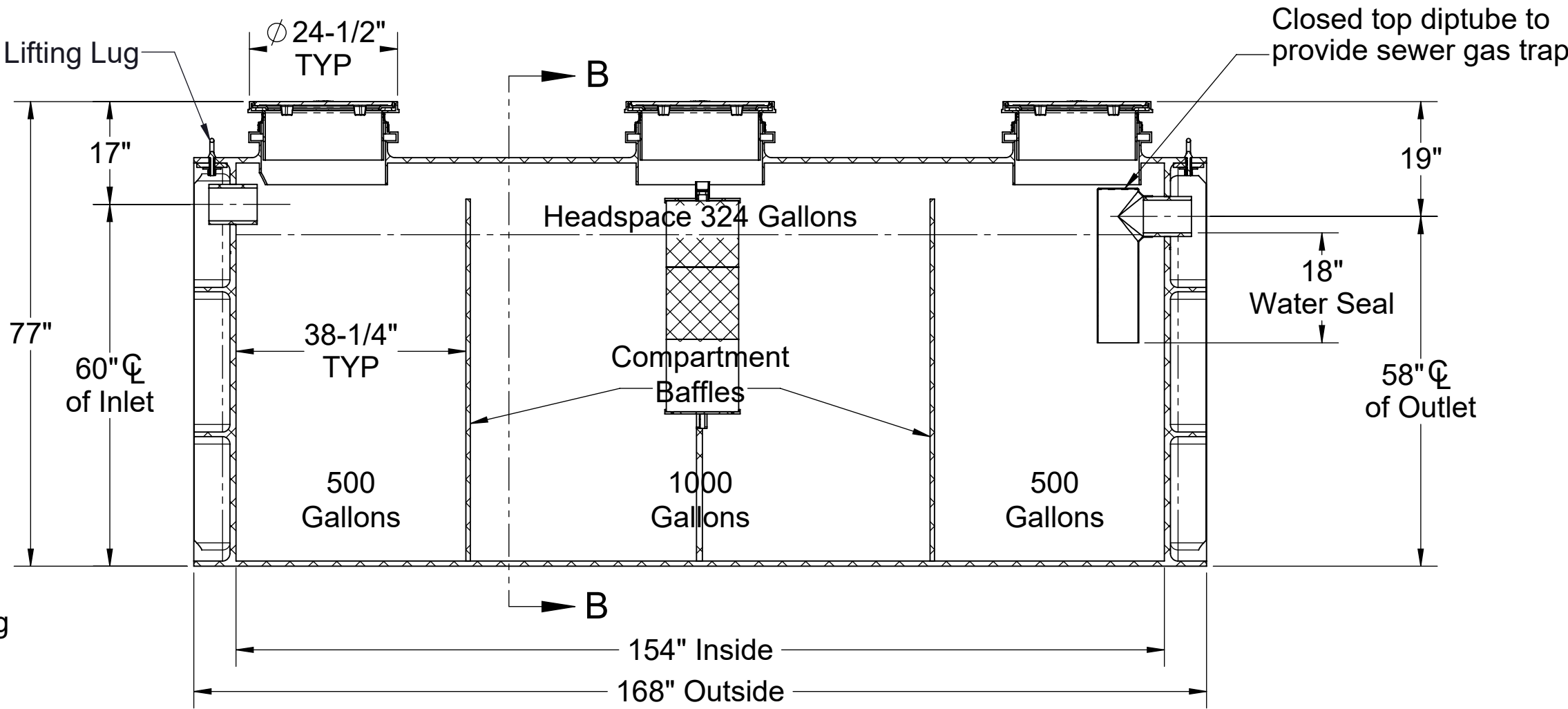
SECTION A-A
