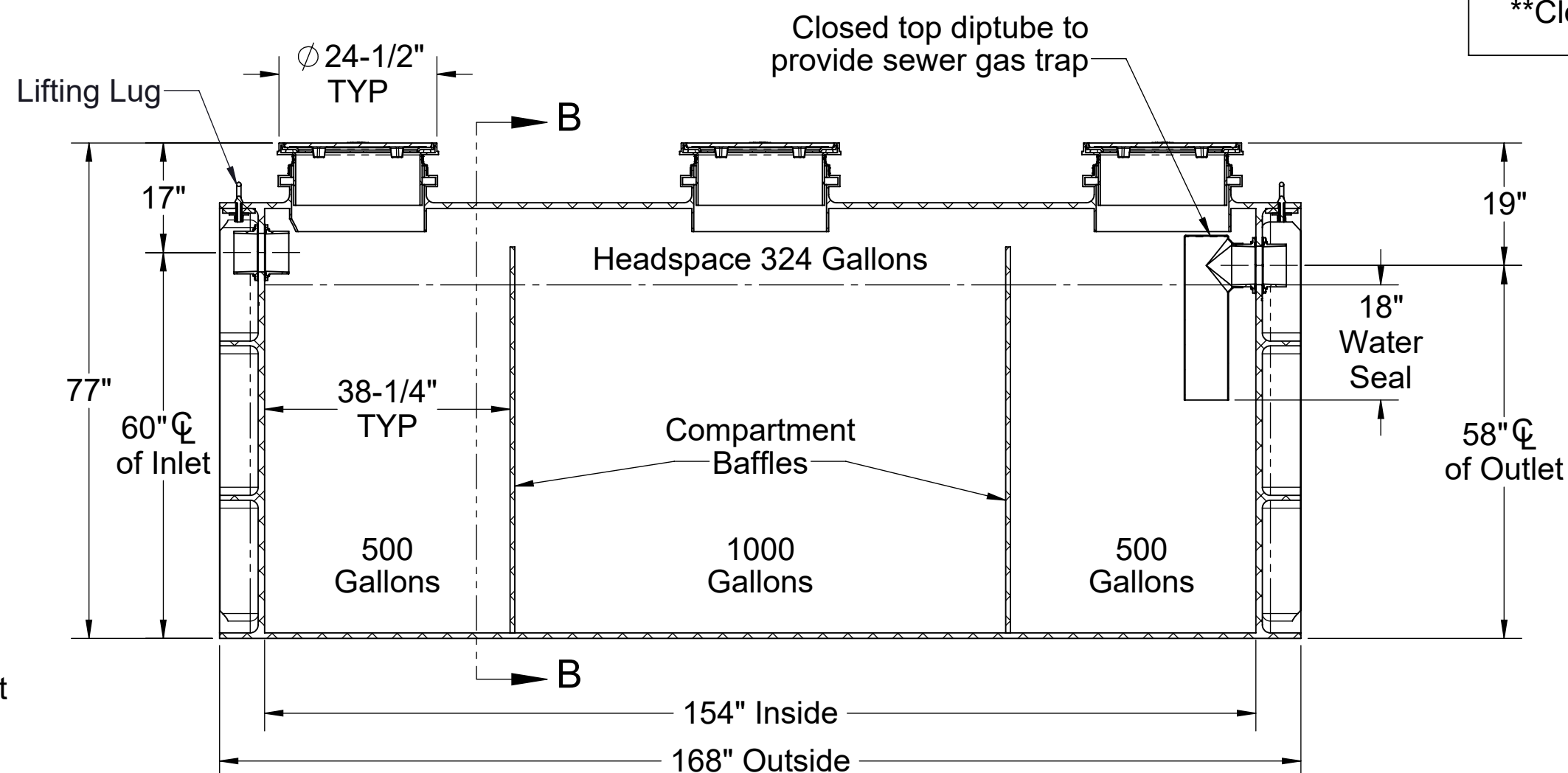
SECTION A-A
