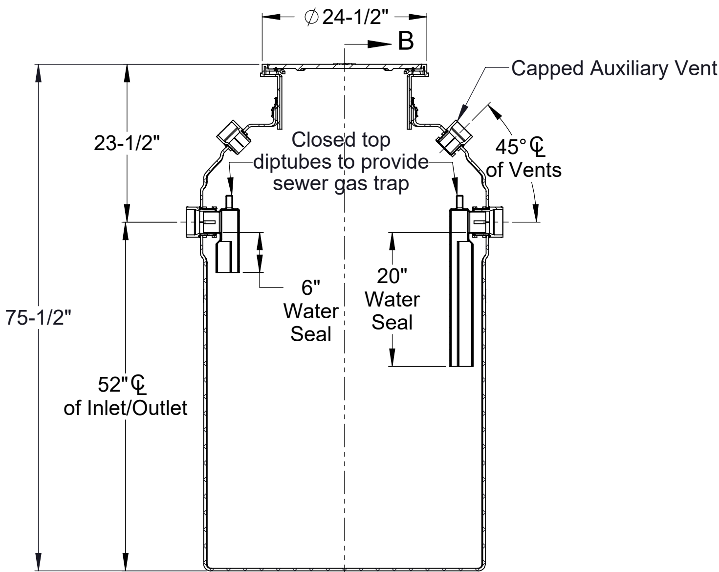
SECTION A-A
