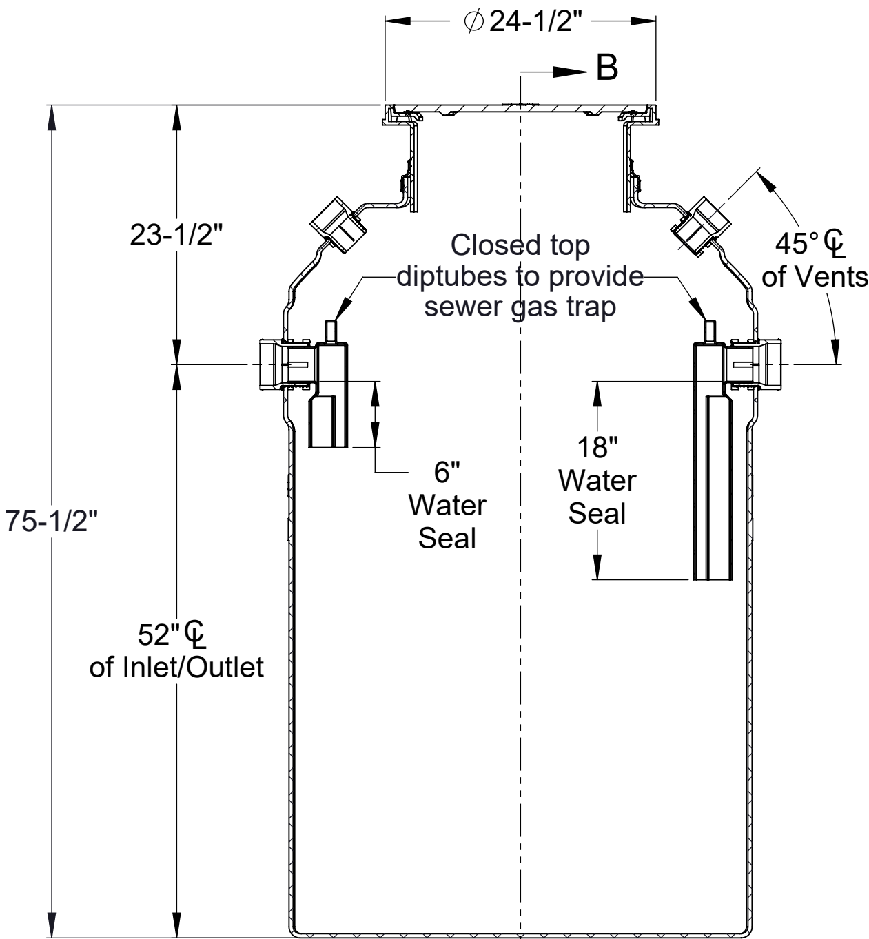
SECTION A-A
