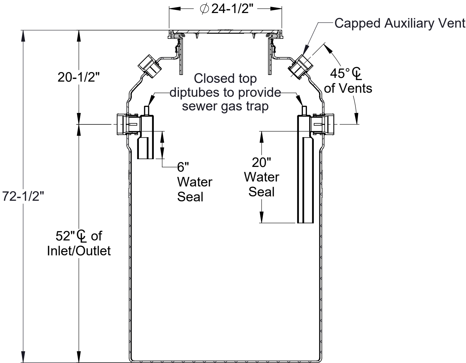
SECTION A-A
