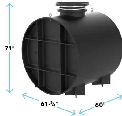
CB-500-G OPTIONS → 24" HDK
