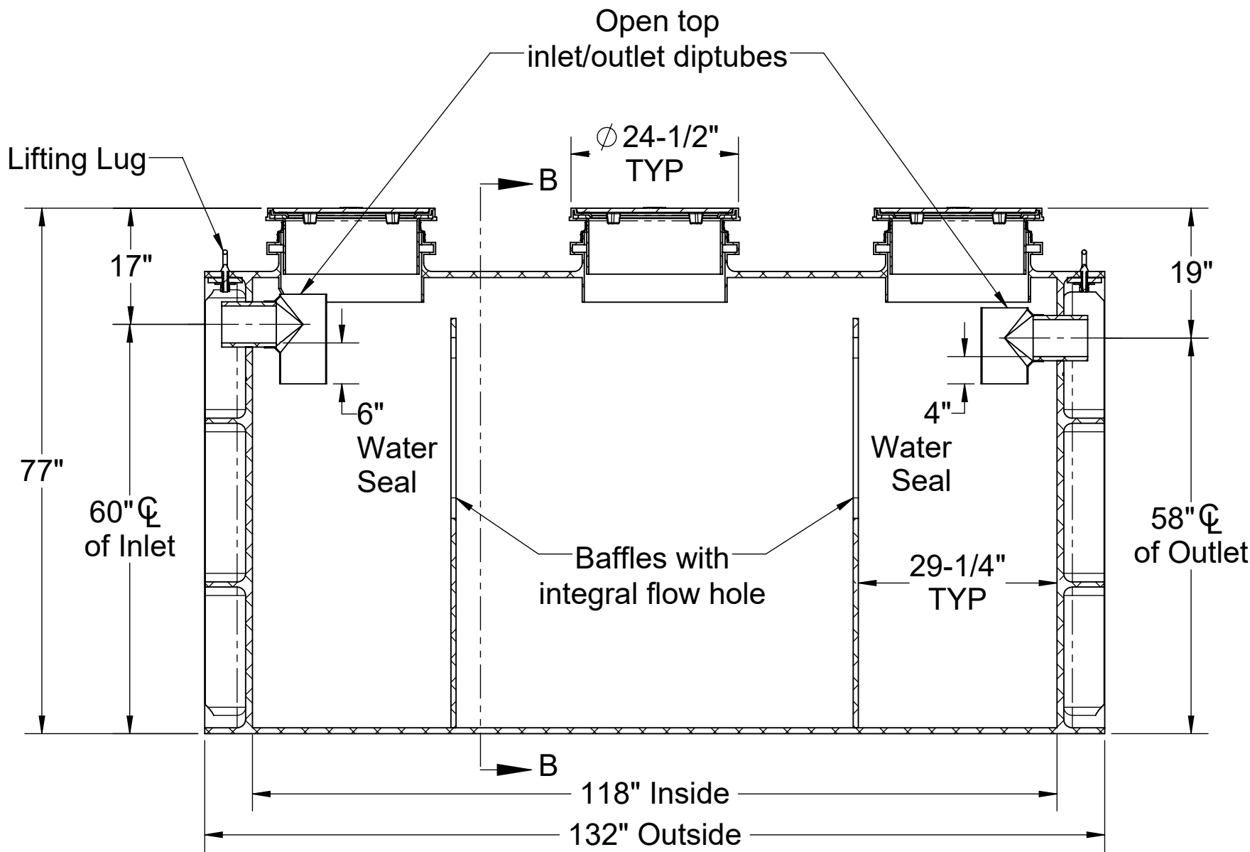
SECTION A-A
