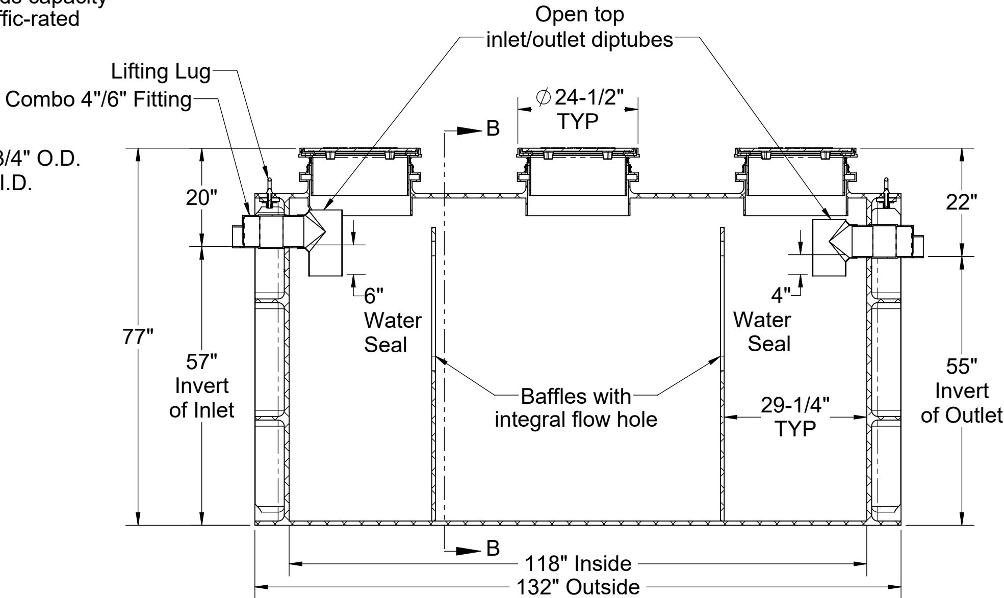
SECTION A-A
