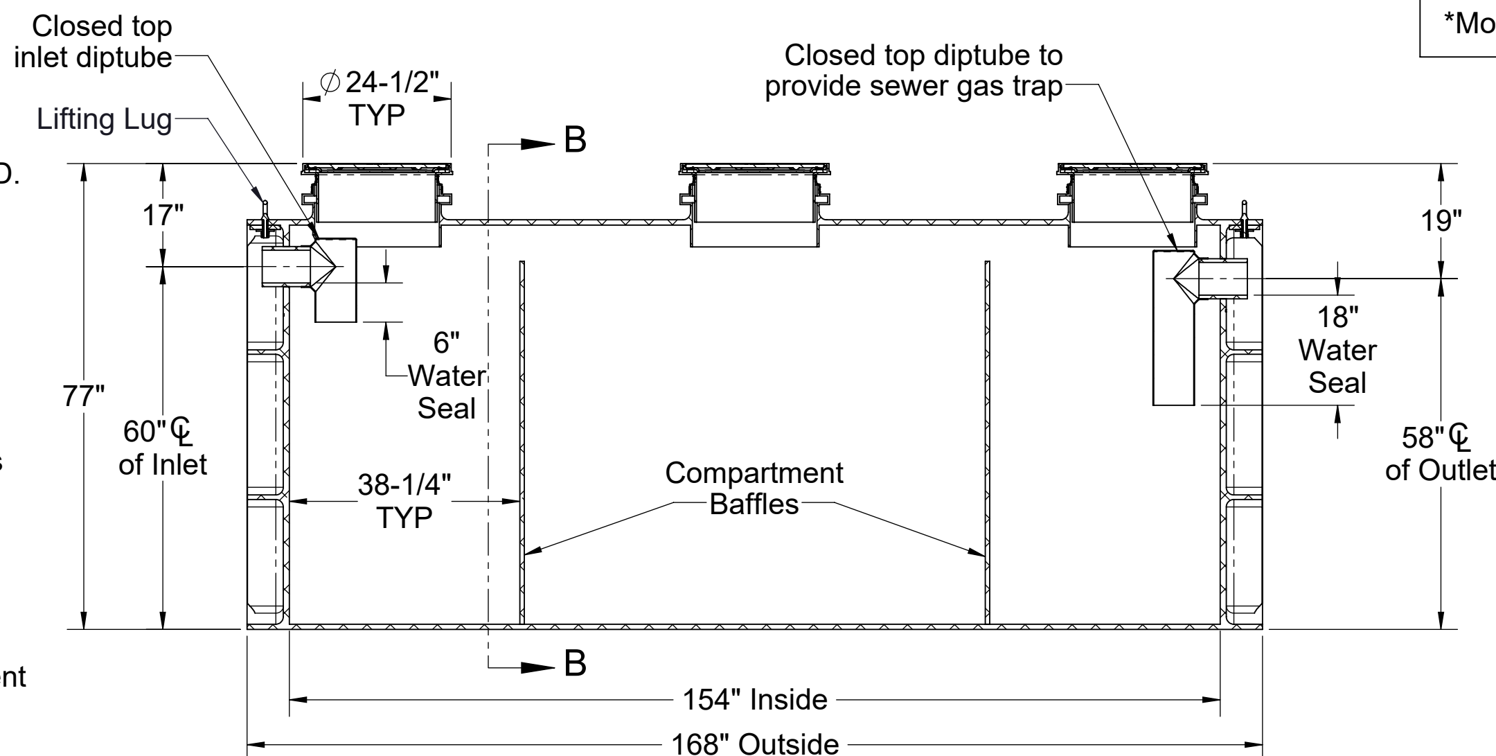
SECTION A-A
