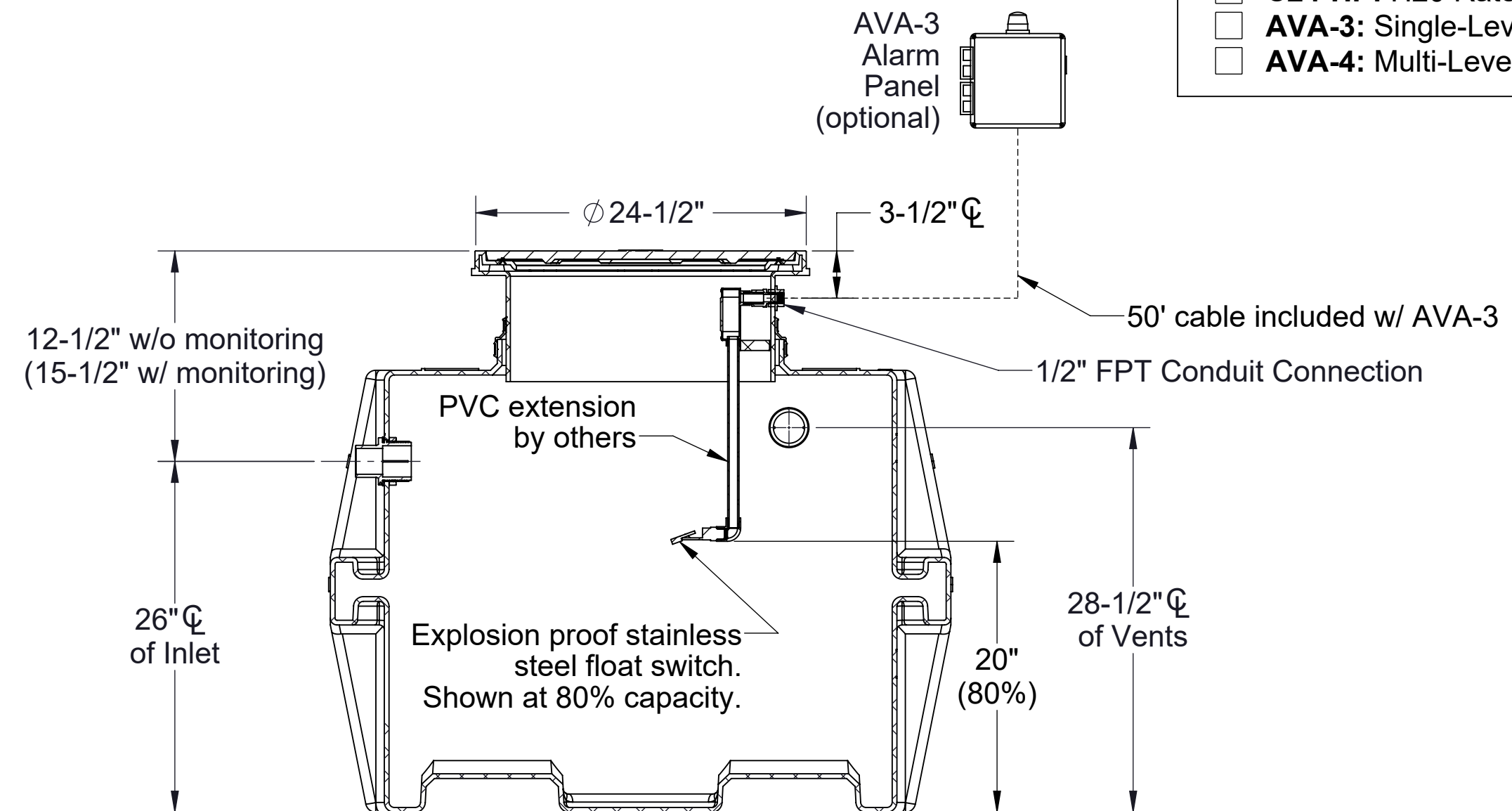
SECTION A-A
