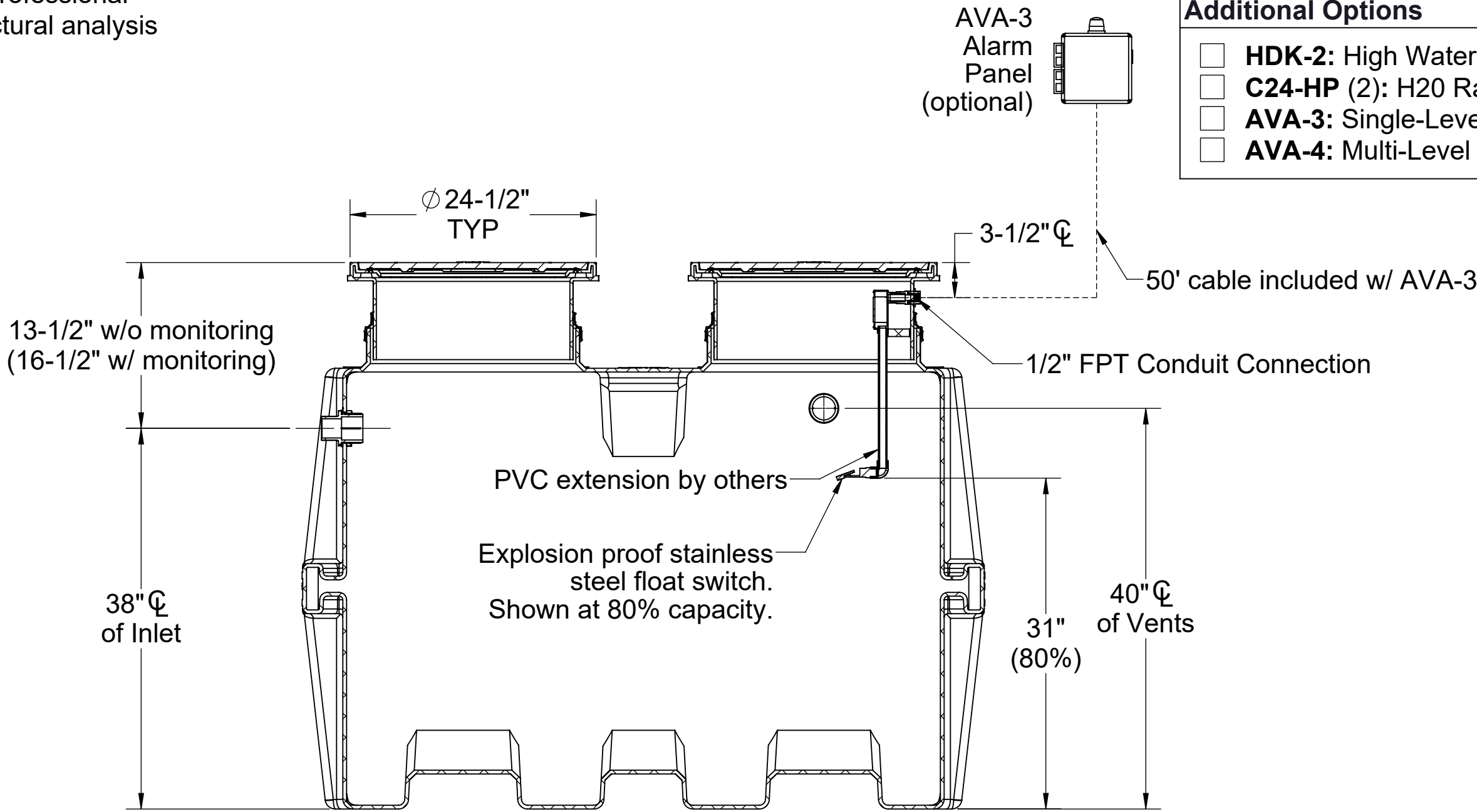
SECTION A-A
