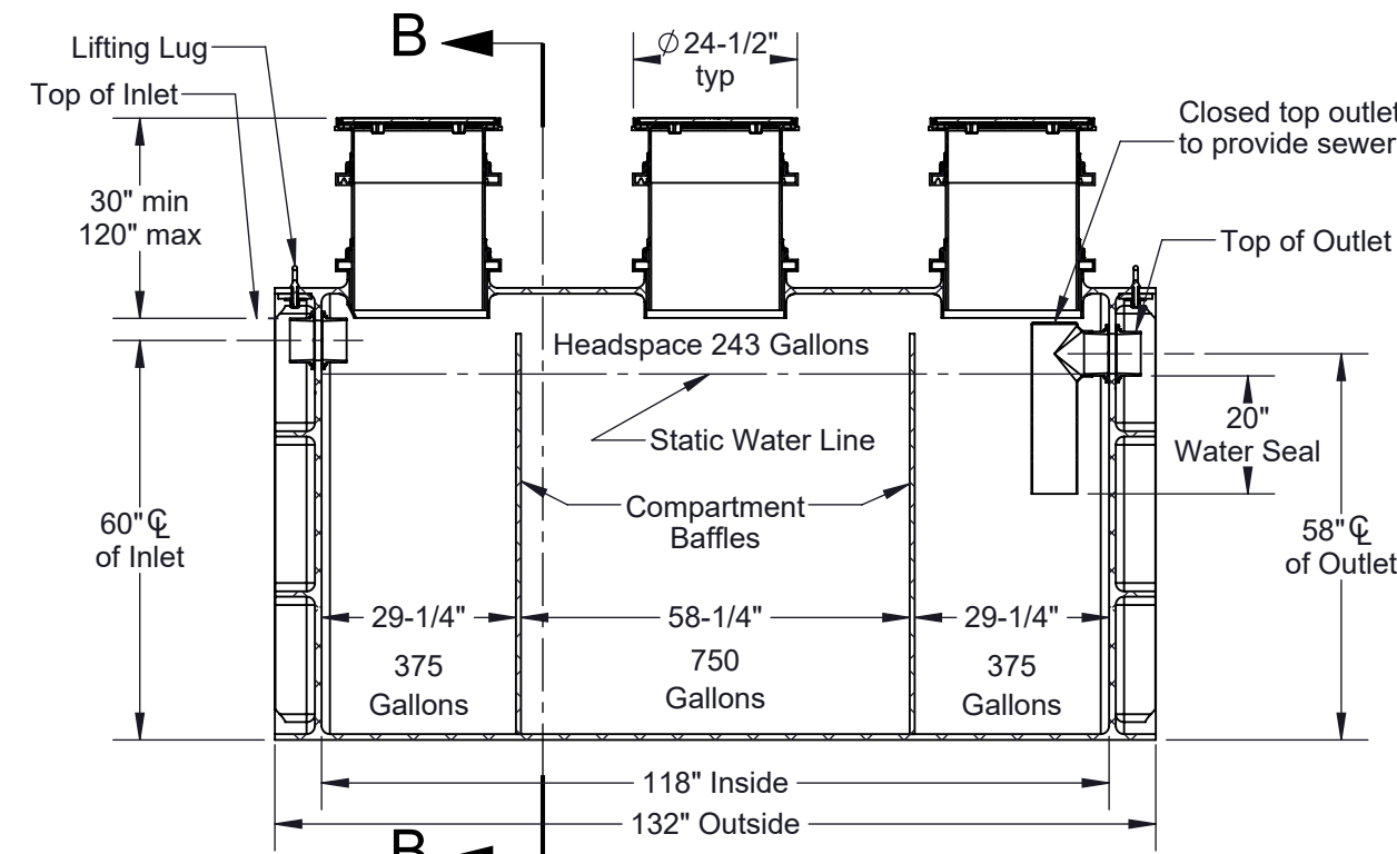
SECTION A-A
