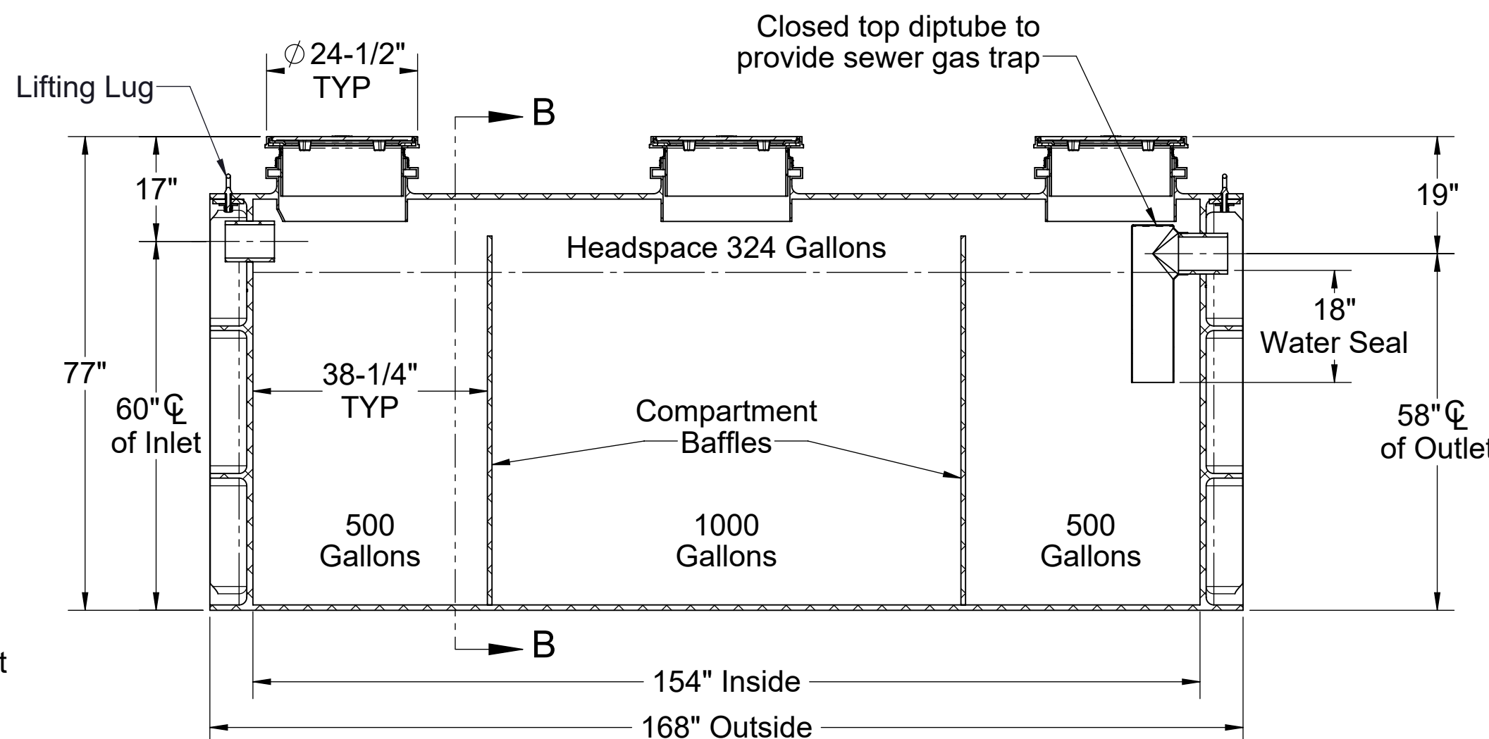
SECTION A-A
