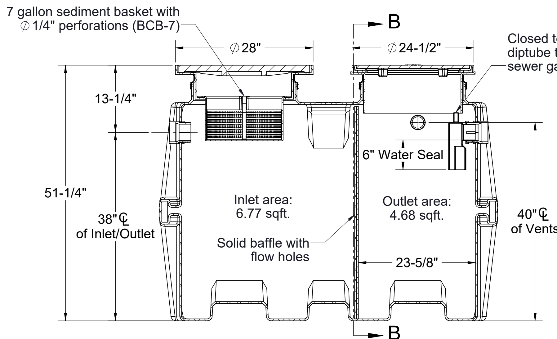
SECTION A-A
