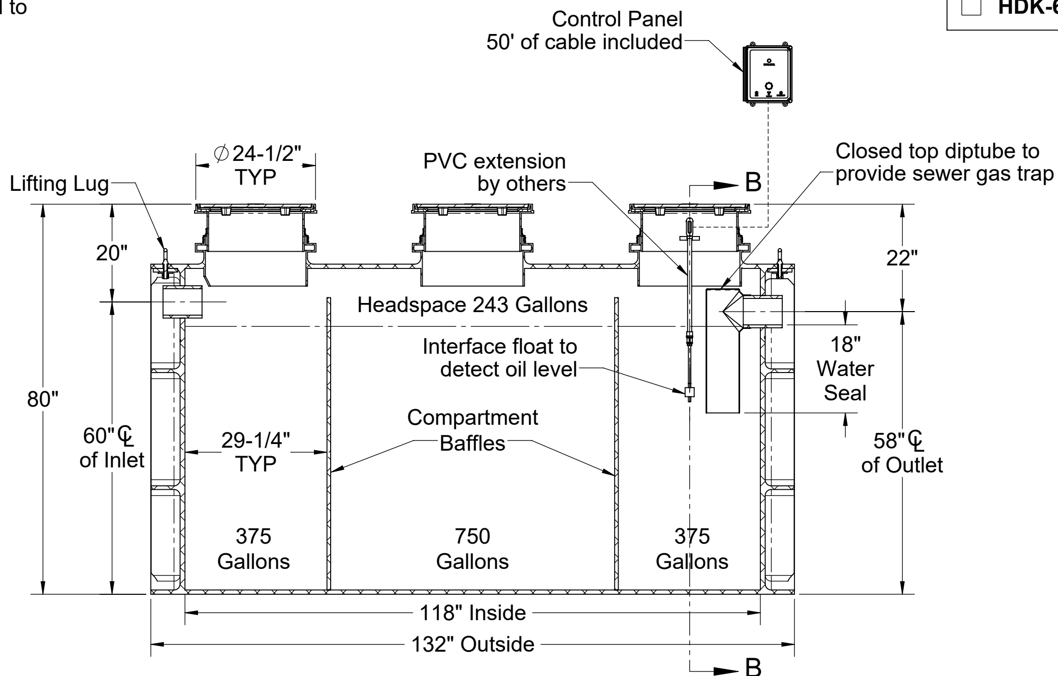
SECTION A-A
