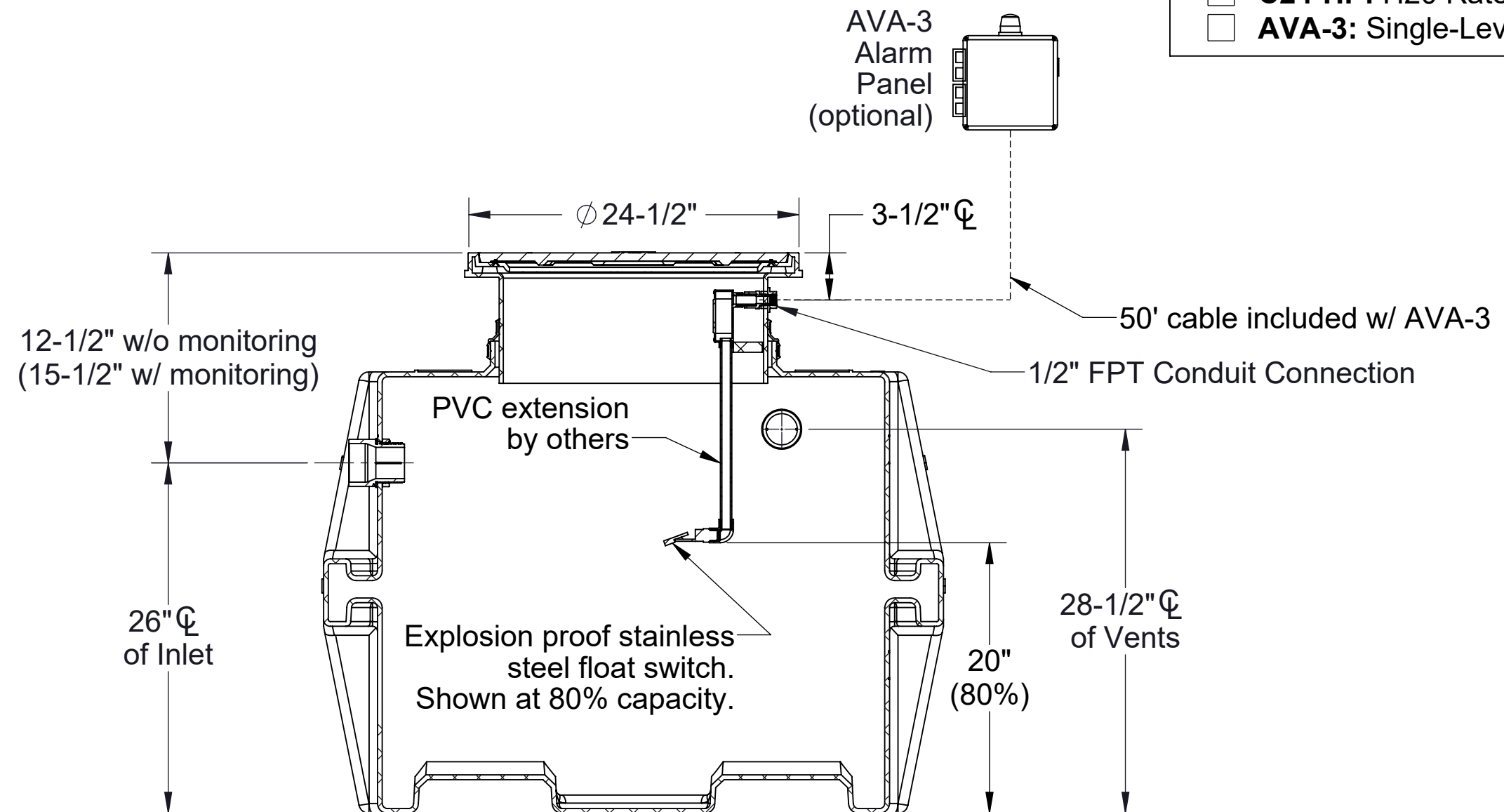
SECTION A-A
