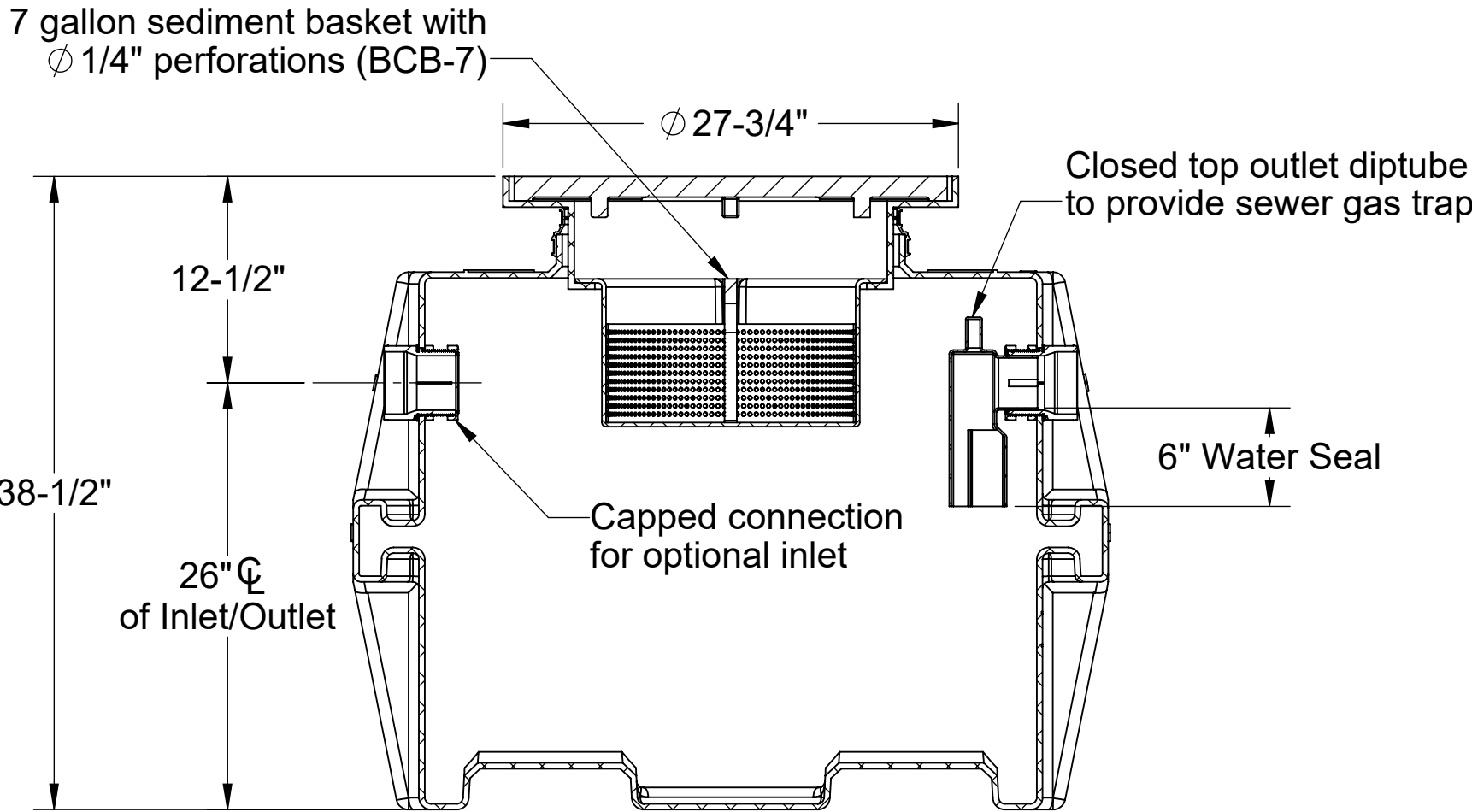
SECTION A-A
