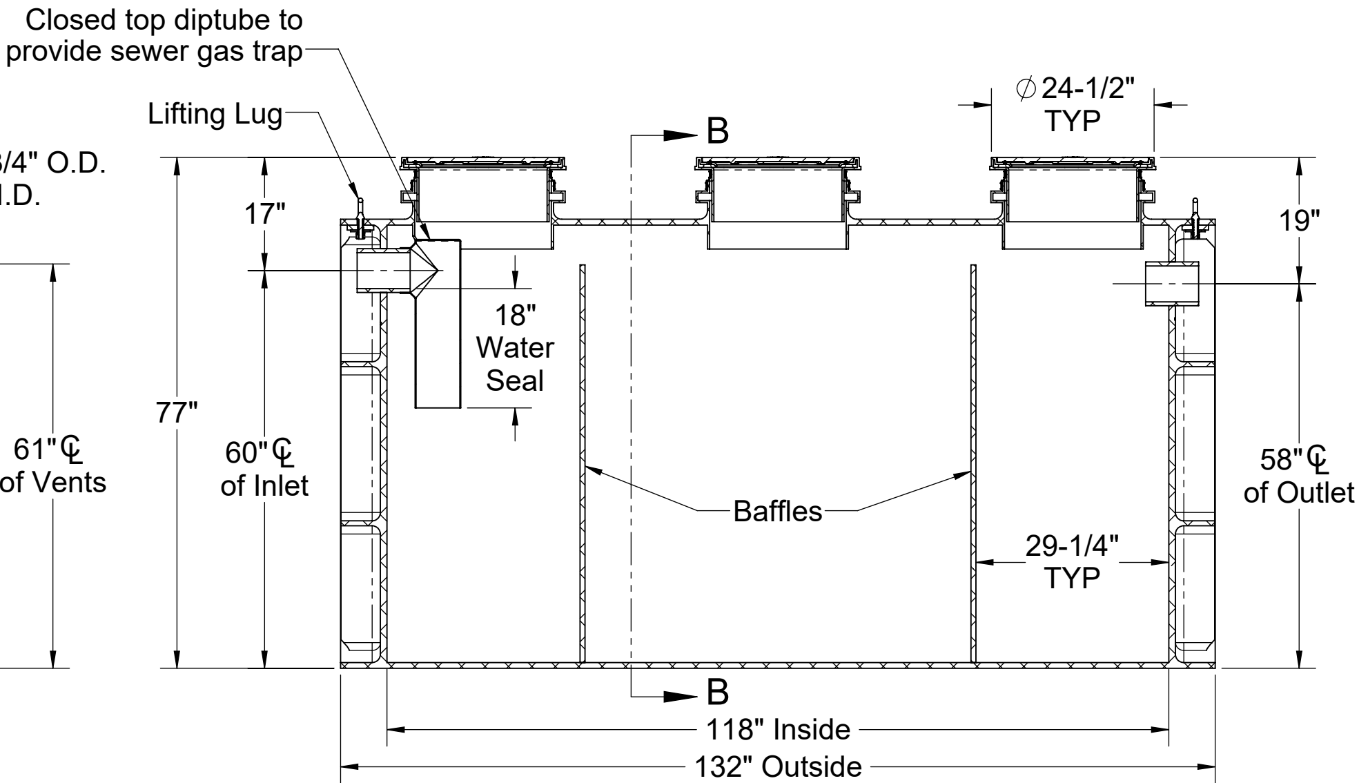
SECTION A-A
