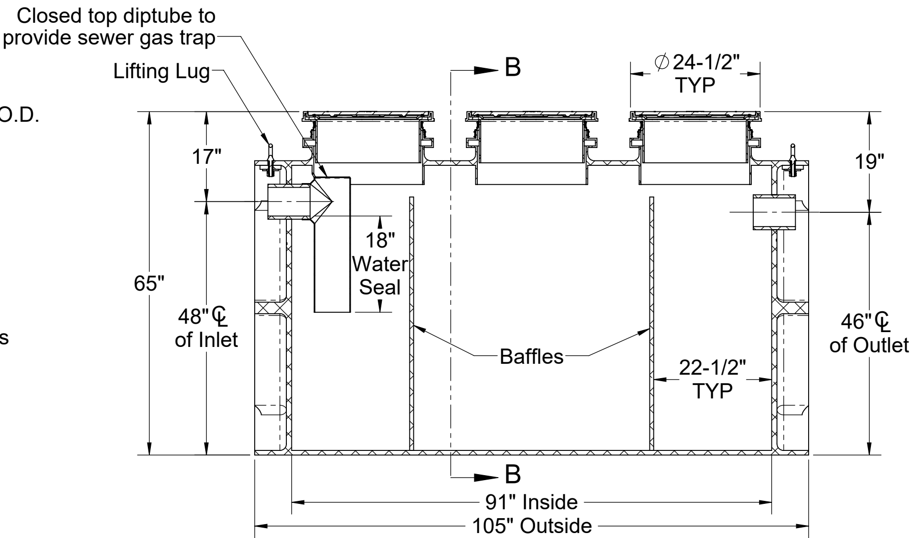
SECTION A-A
