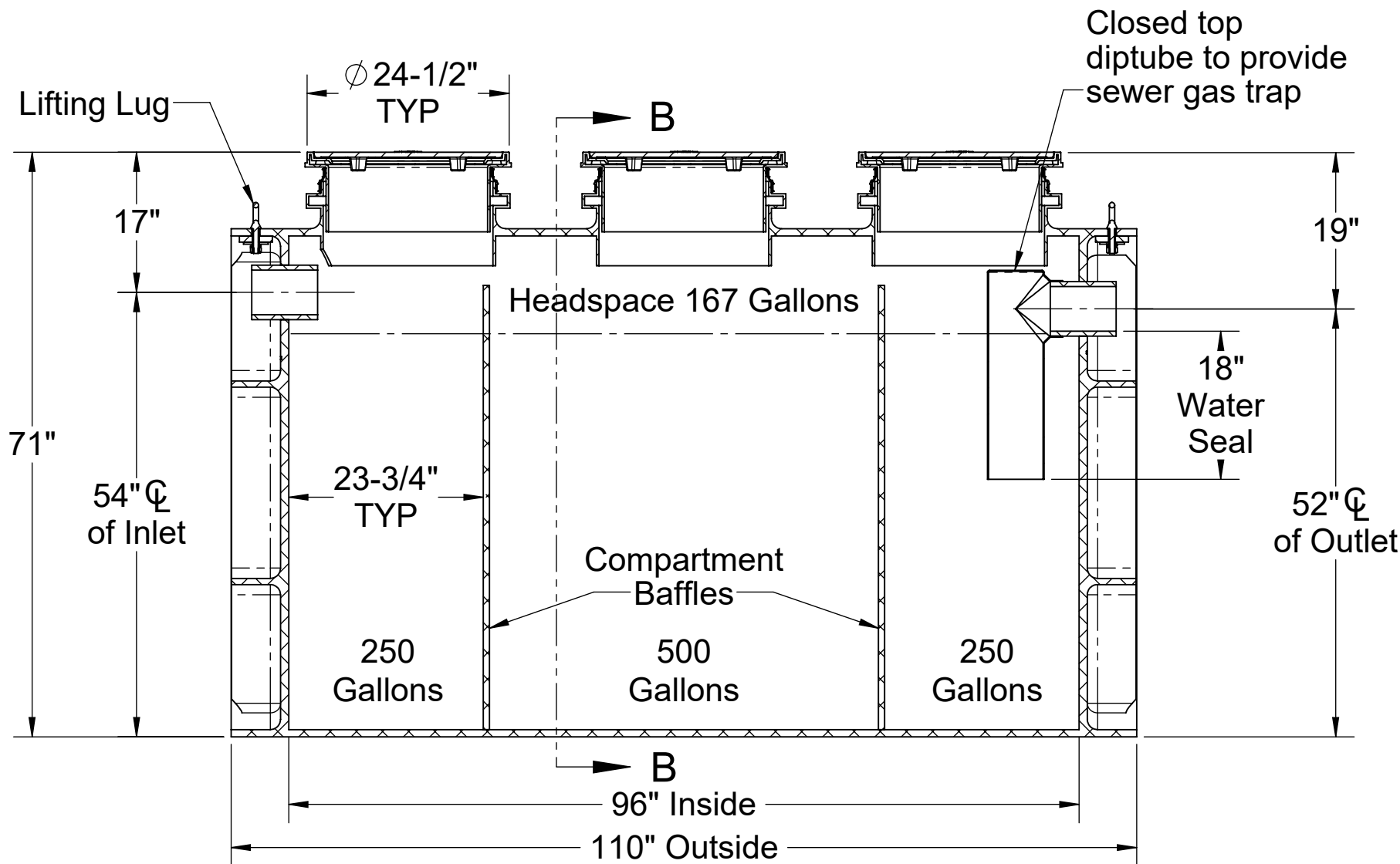
SECTION A-A
