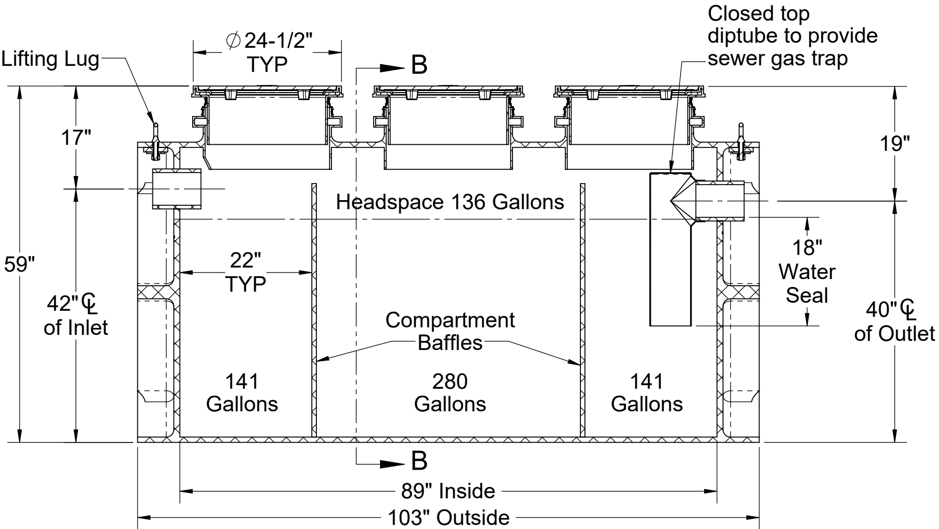
SECTION A-A
